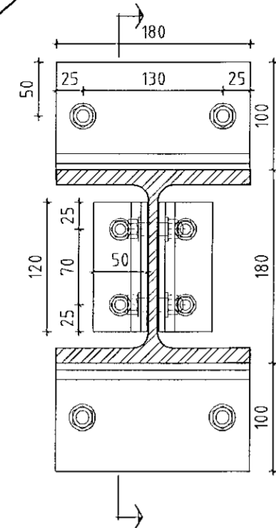
Sérmynd T2-1 1:5
