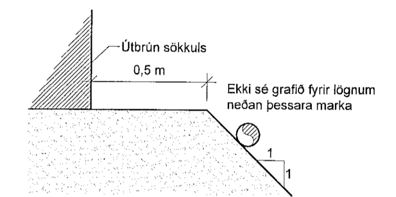
Leqa lagna við hús 1:20
