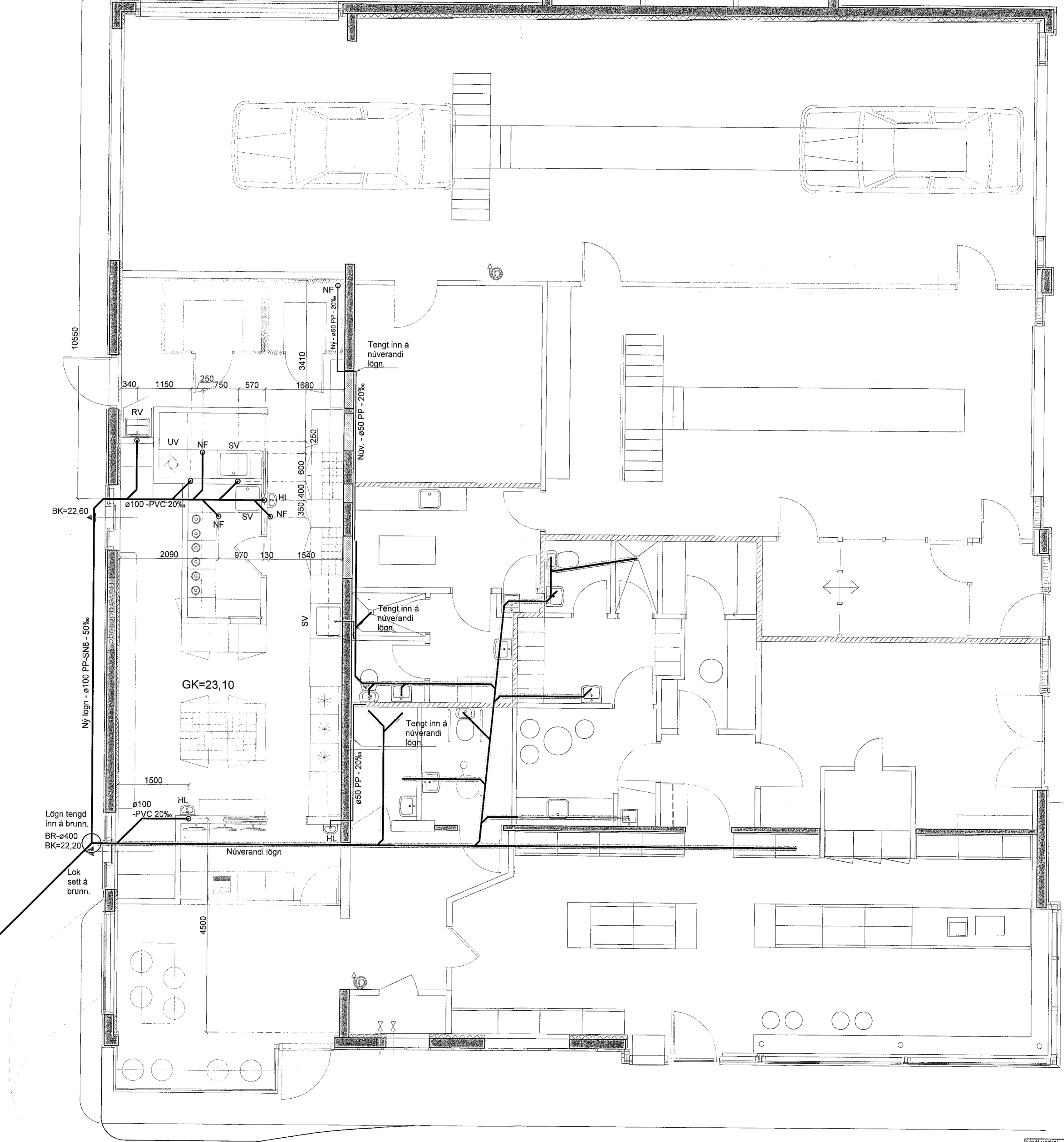
Lagnir í sökkli Mkv. 1:50
