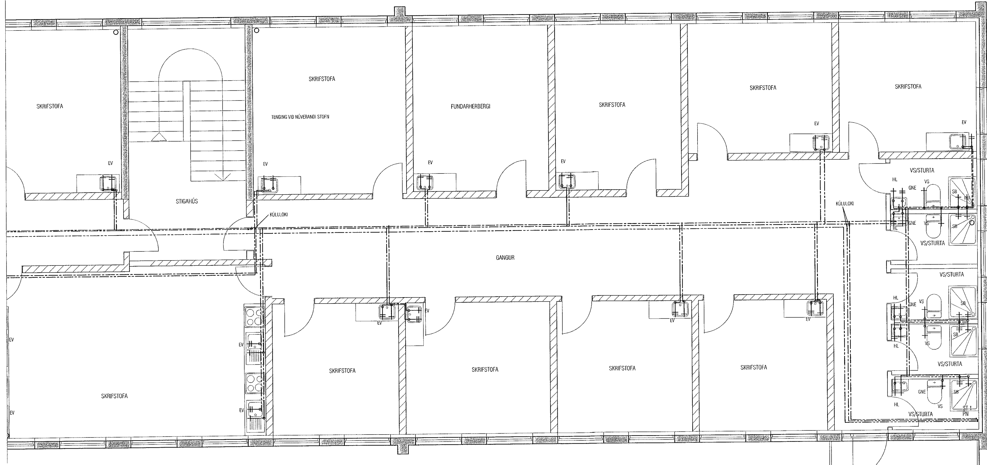
GRUNNMYND 3. HÆÐAR TIL HÆGRI, NEYSLUVATN MKV. 1:50
