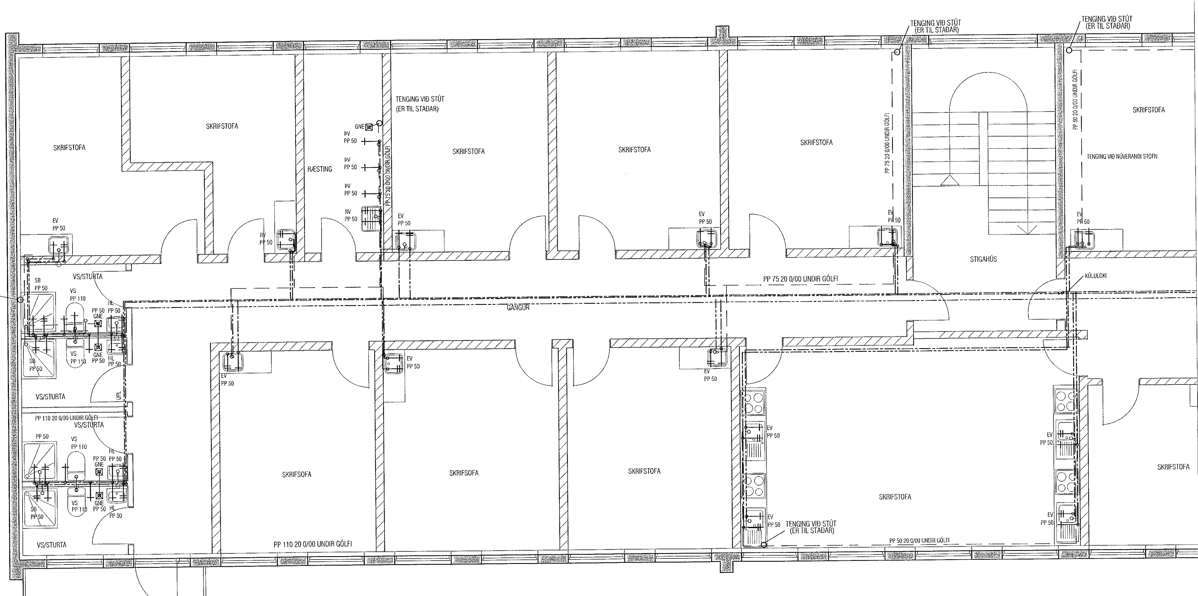
GRUNNMYND 3. HÆÐAR TIL VINSTRI, NEYSLUVATN MKV. 1:50
