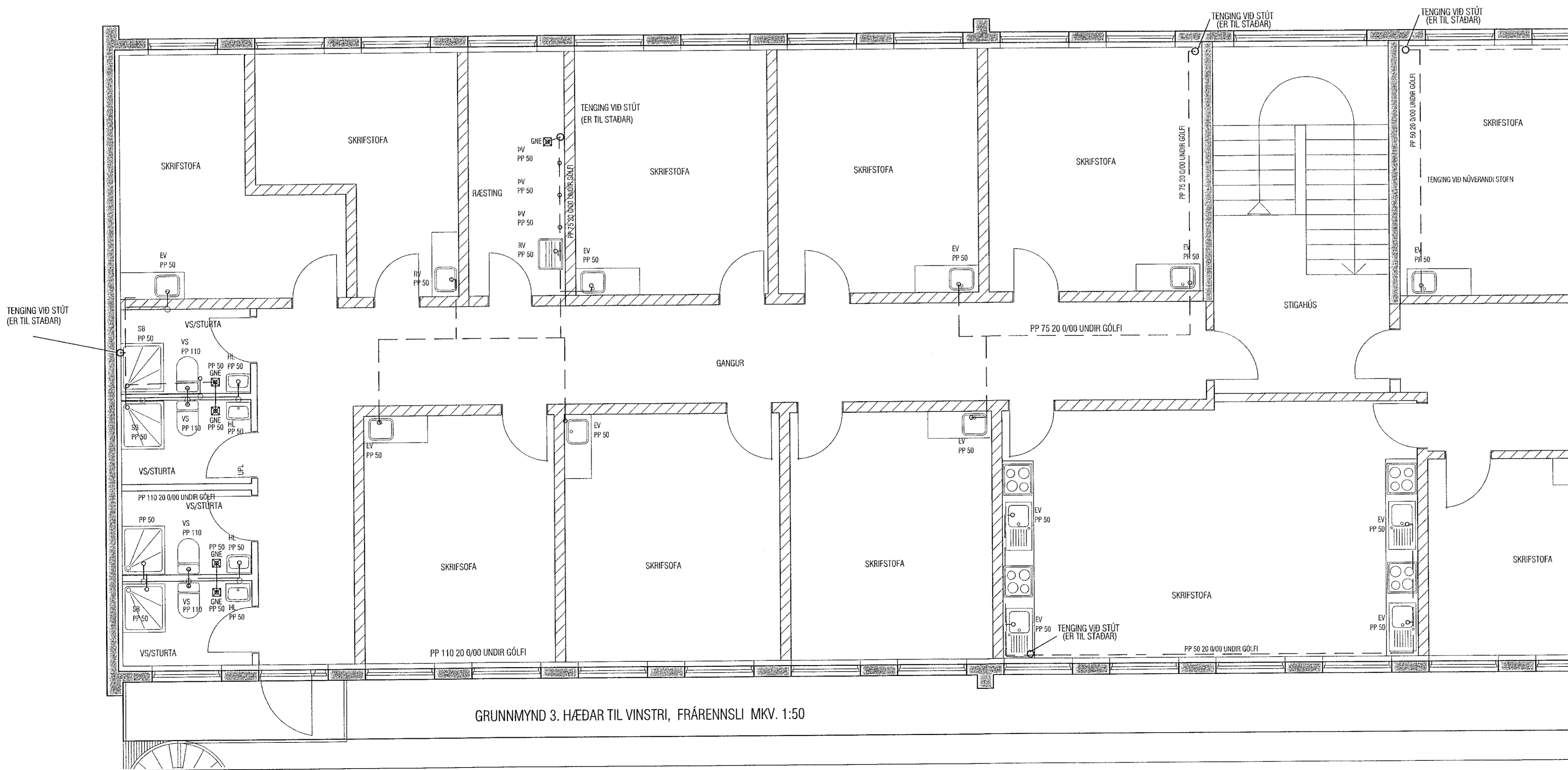
GRUNNMYND 3. HÆÐAR TIL HÆGRI, FRÁRENNSLI MKV. 1:50
