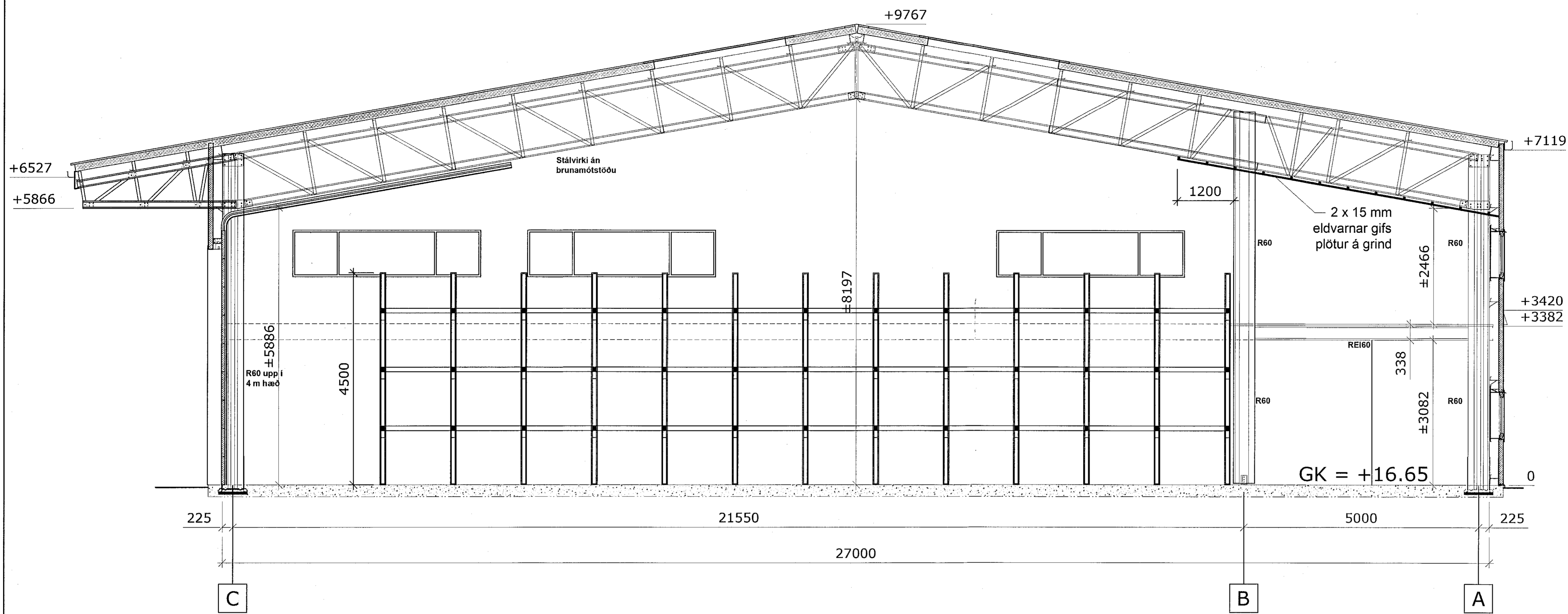
Snið A - A.
