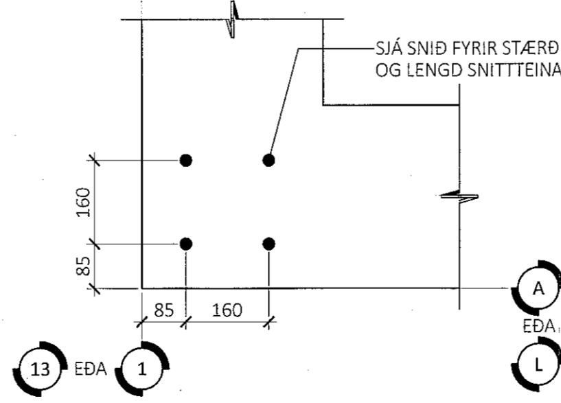
INNSTEYPTIR SNITTEINAR Á HORNUM - M1:5:
