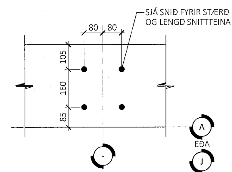
INNSTEYPTIR SNITTEINAR Á LANGHLÍÐUM - M1:10:
