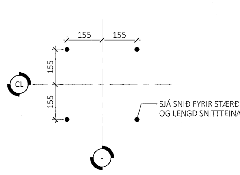
INNSTEYPTIR SNITTEINAR FYRIR SÚLUR Í MÁTLÍNU CL - M1:5:
