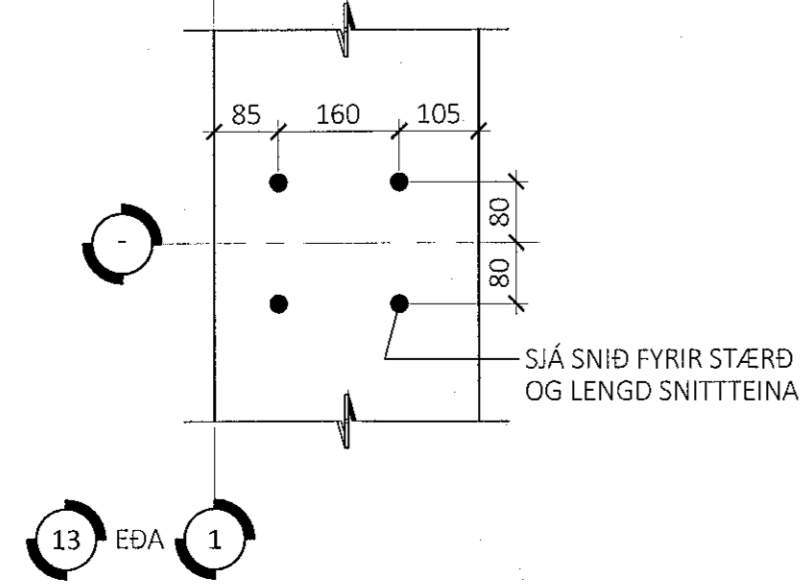
INNSTEYPTIR SNITTEINAR Á SKAMMHLÍÐUM - M1:5:
