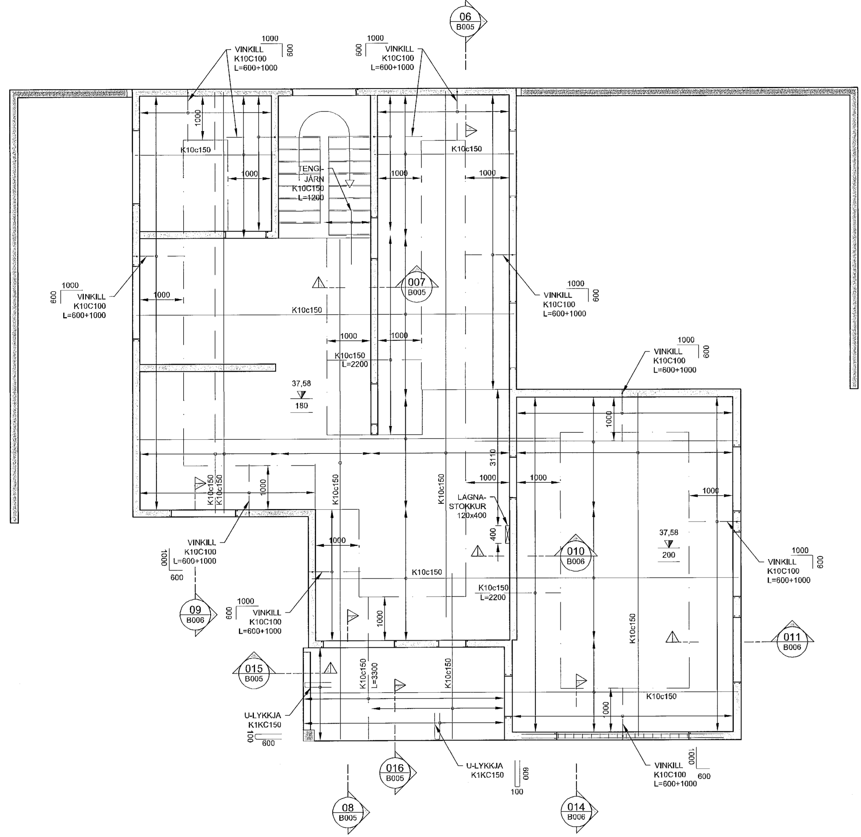
GRUNNMYND PLATA 1.HÆÐ 1:50 (A2)
