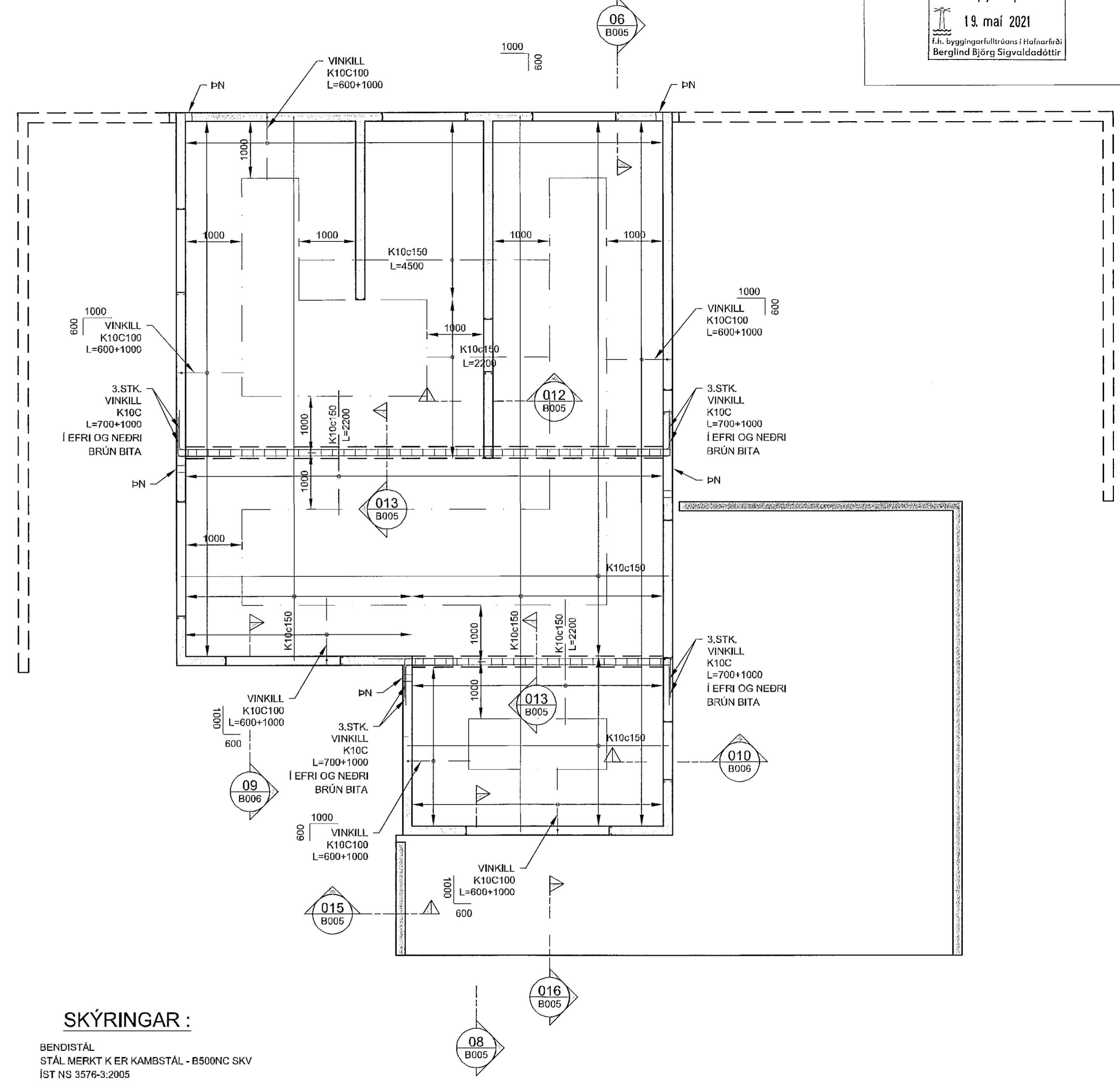
GRUNNMYND PLATA 2.HÆÐ 1:50 (A2)
