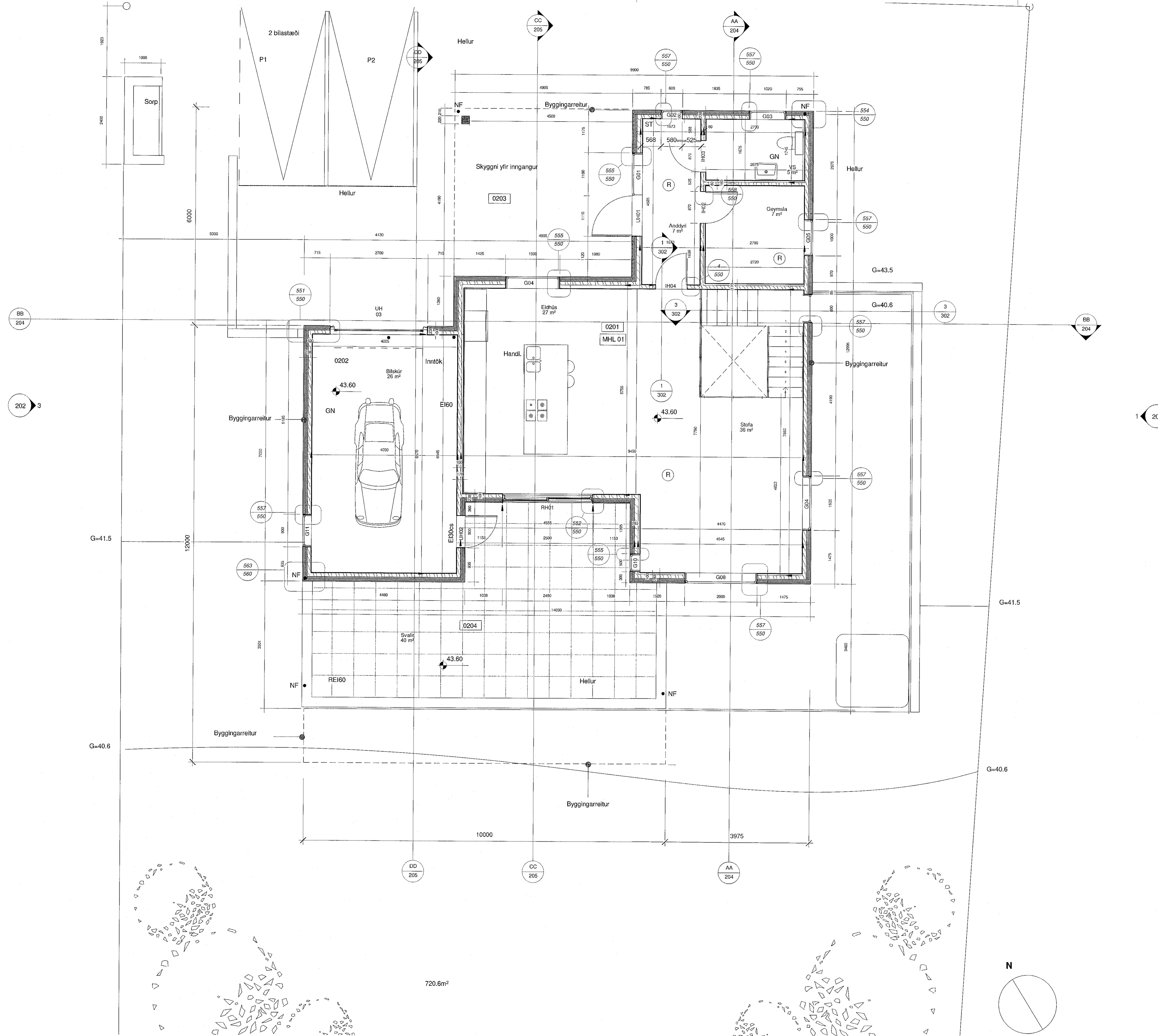
2.Hæð mkv: 1 : 50
