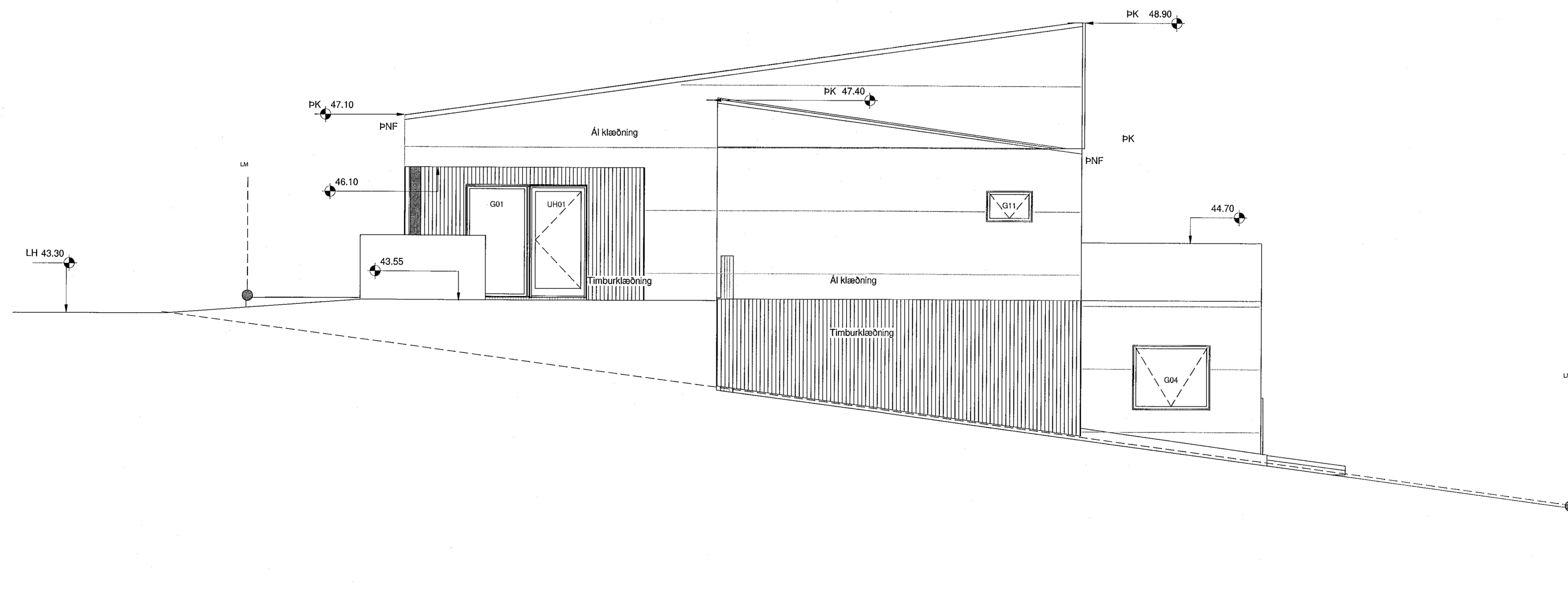
Útlit vestur mkv: 1 : 50
