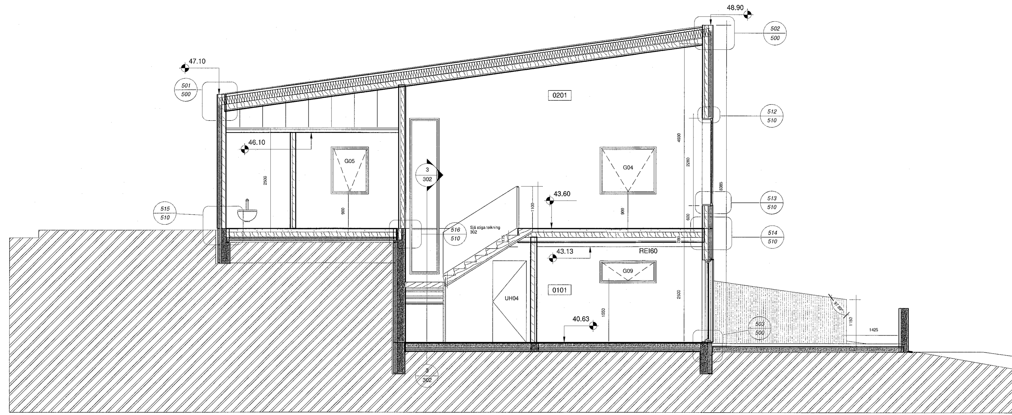
Sneið AA mkv: 1 : 50
