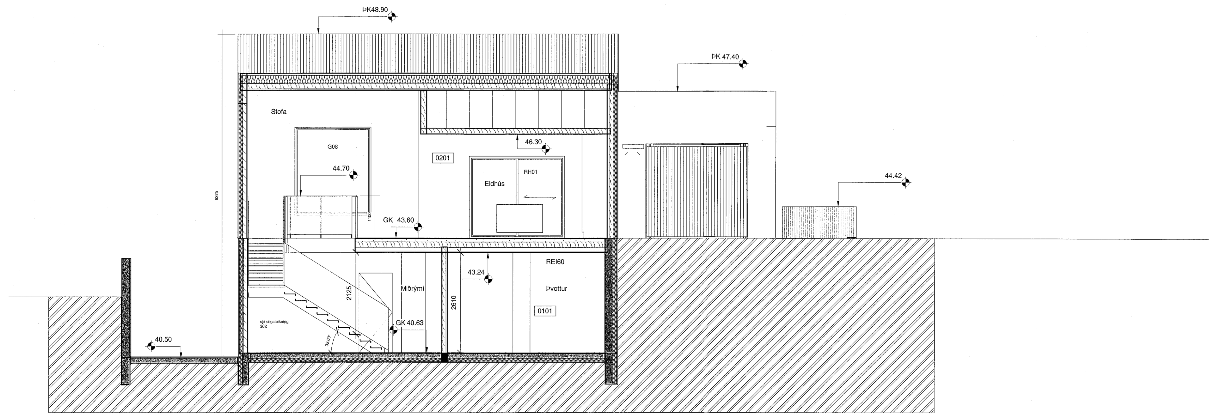
Sneið BB mkv: 1 : 50
