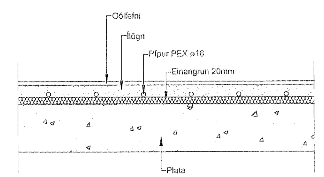
Snið í gólfhita M 1:10
