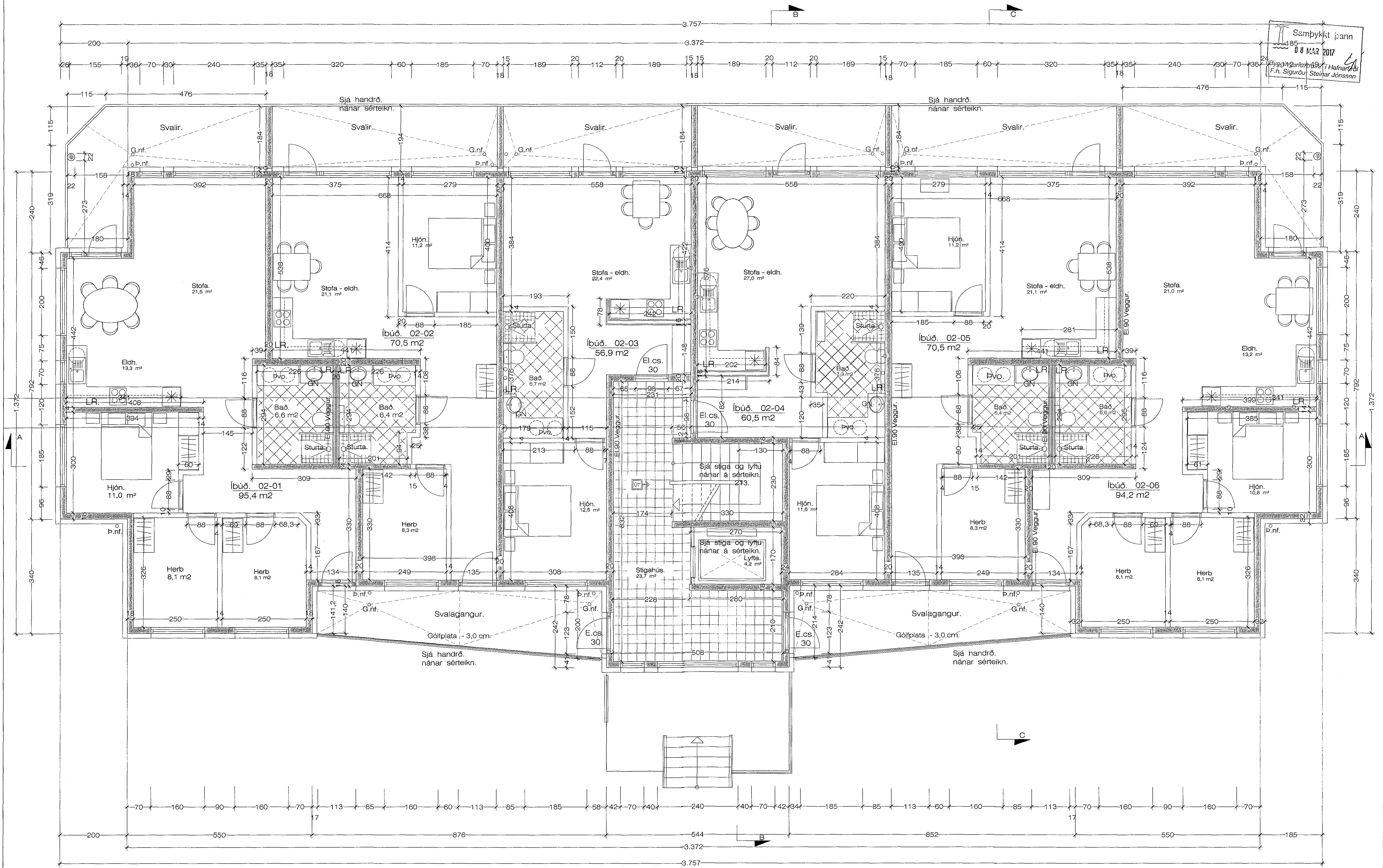
Grunnmynd 3. hæð. Hús Nr. 1 1 : 50 Stærð. 490,0 m 2
