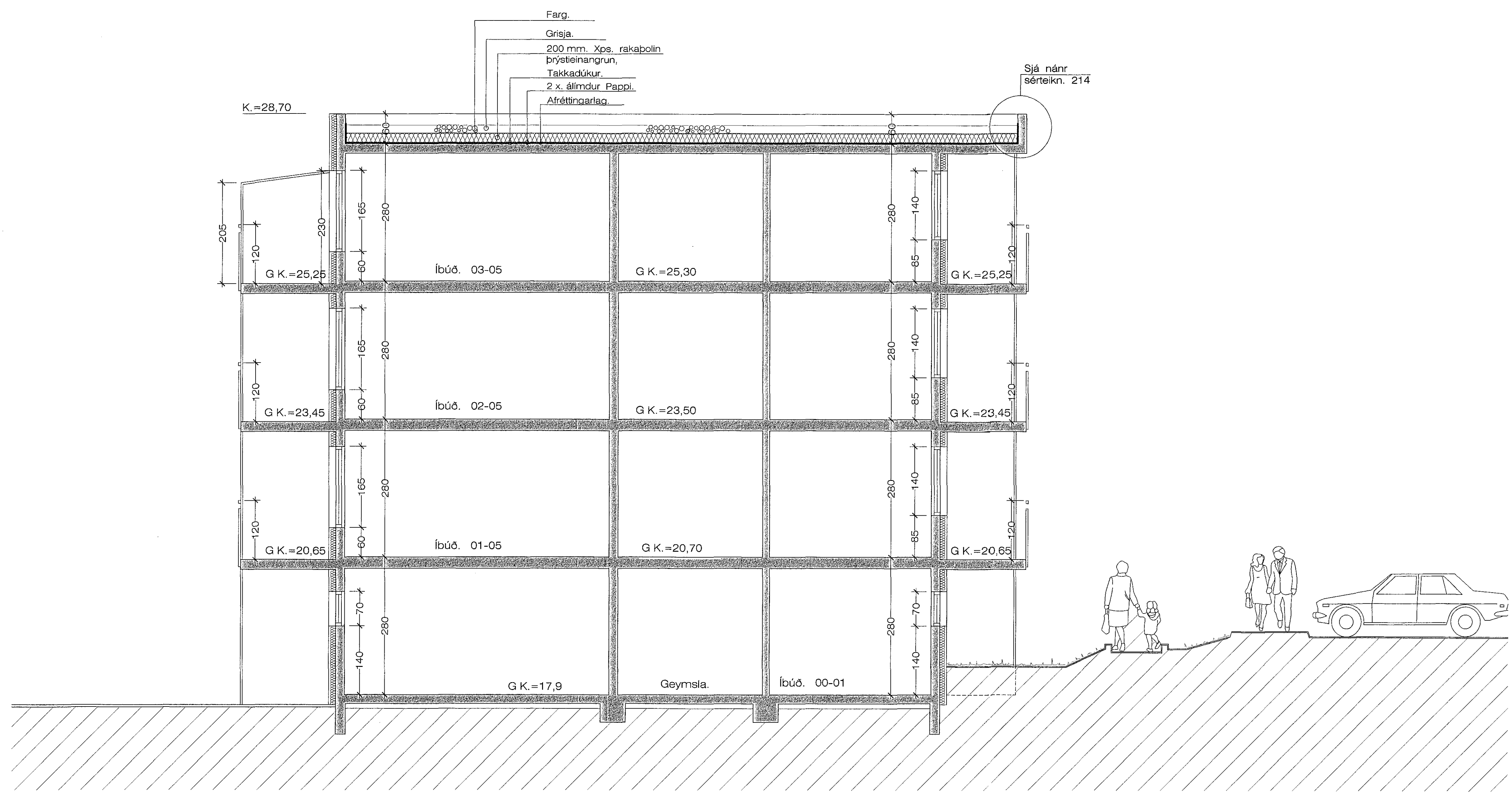
Sneiðing C - C Hús Nr. 1 1 : 50
