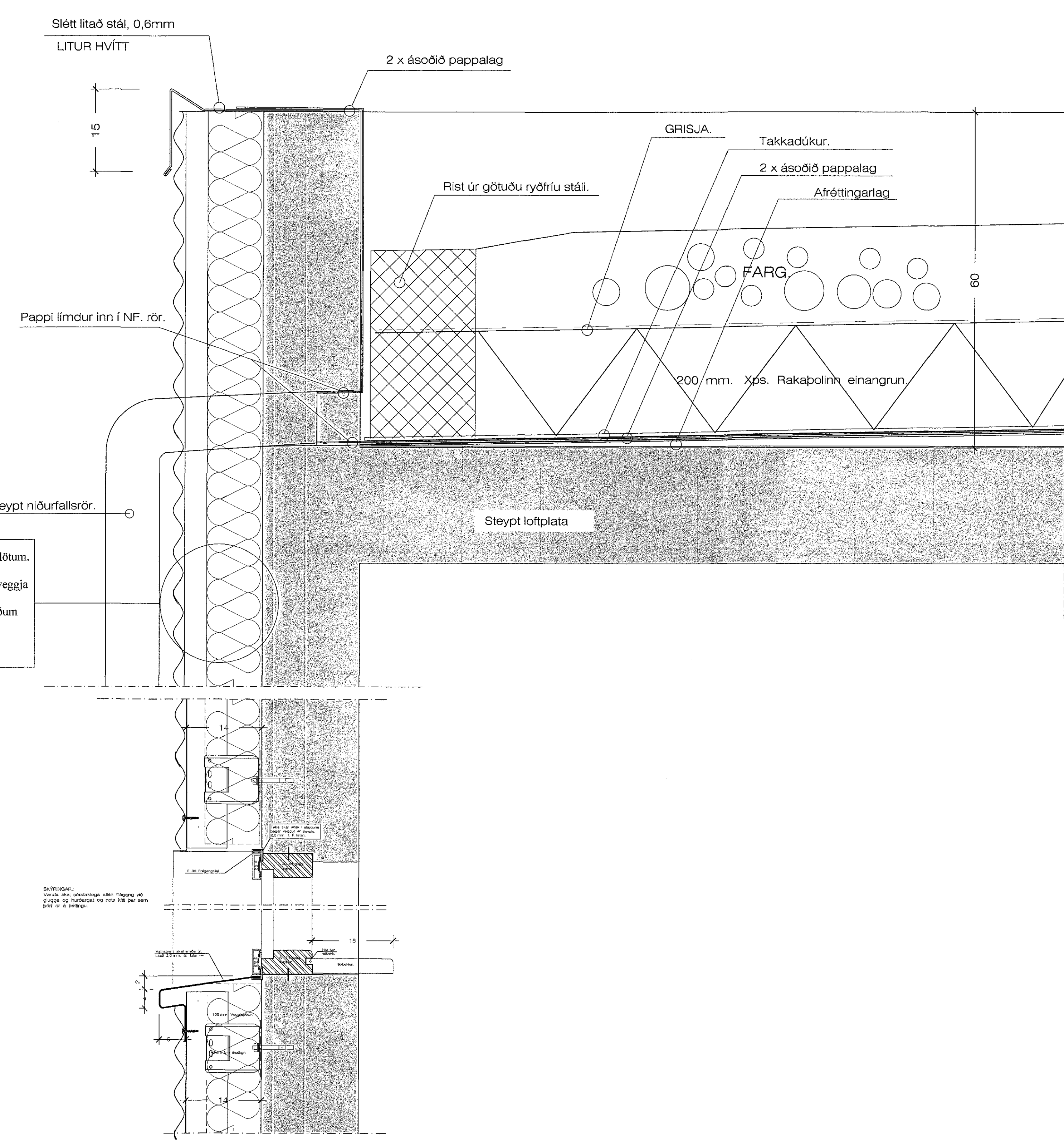
Pakkantar. á flötu þaki. 1:5
