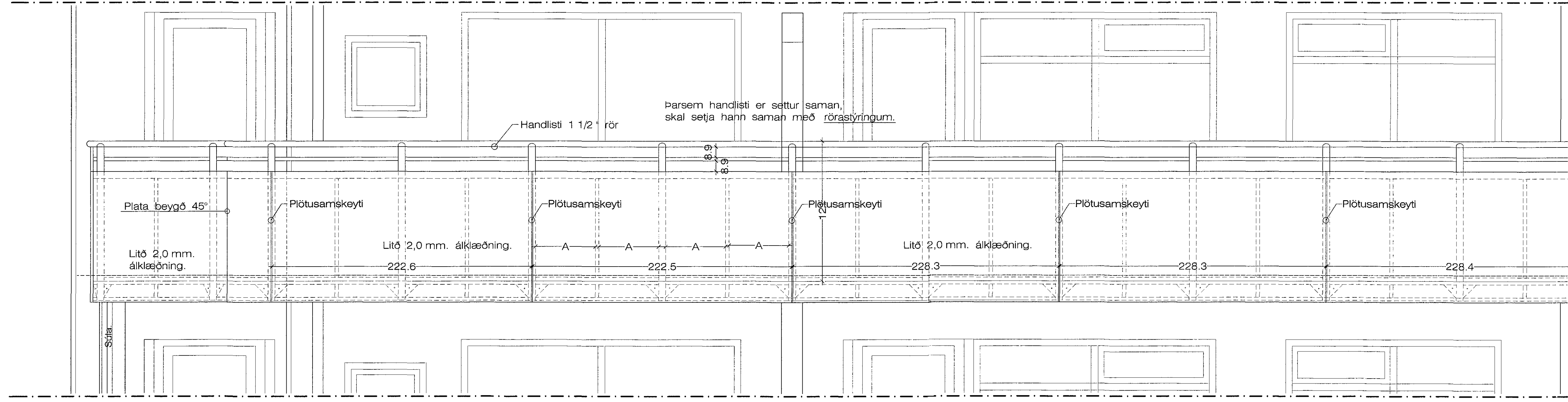
Séð framaná Svalahandrið á baklið hússins. 1:20
