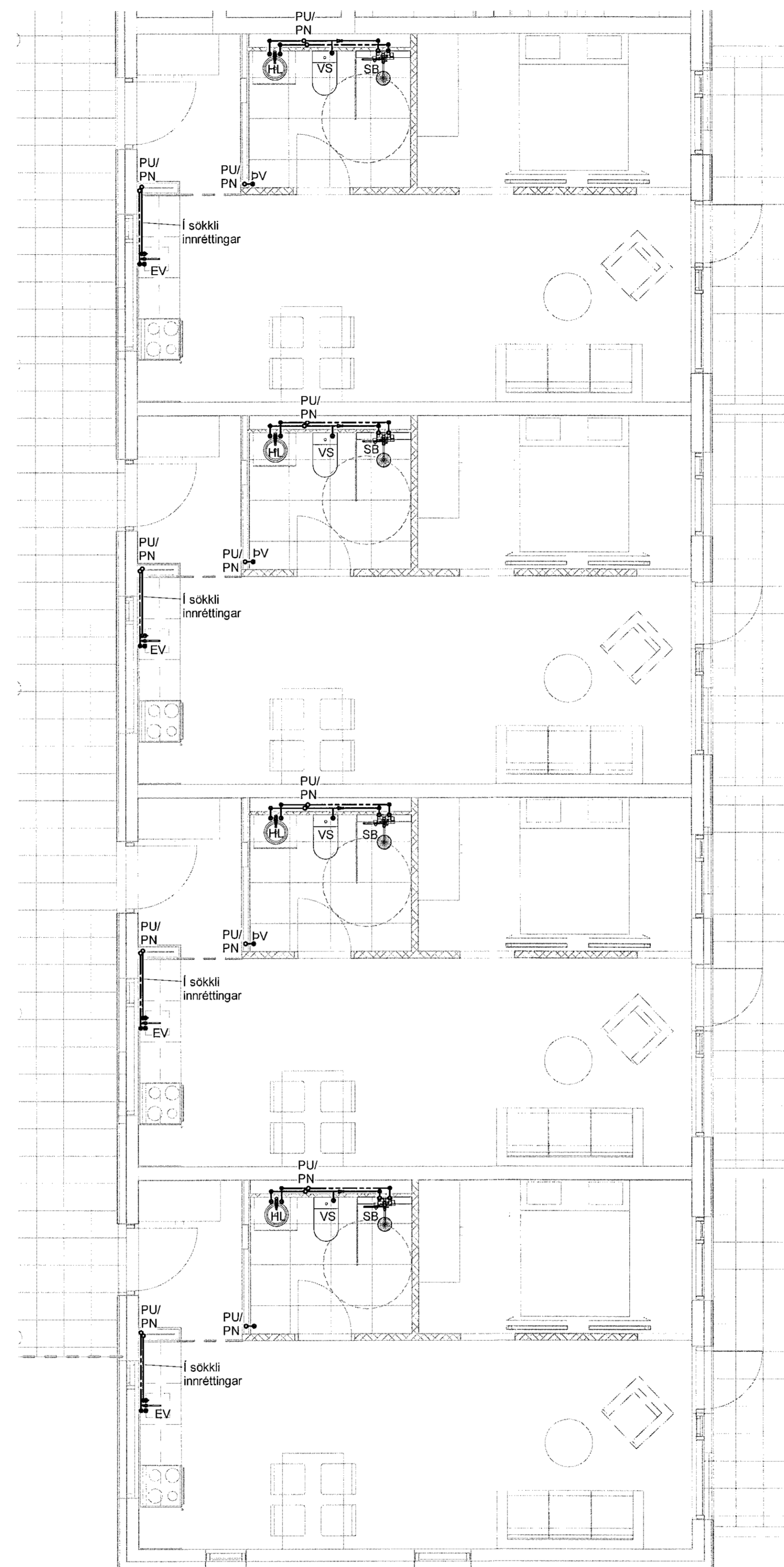
1 1. hæð - 4 1 : 50
