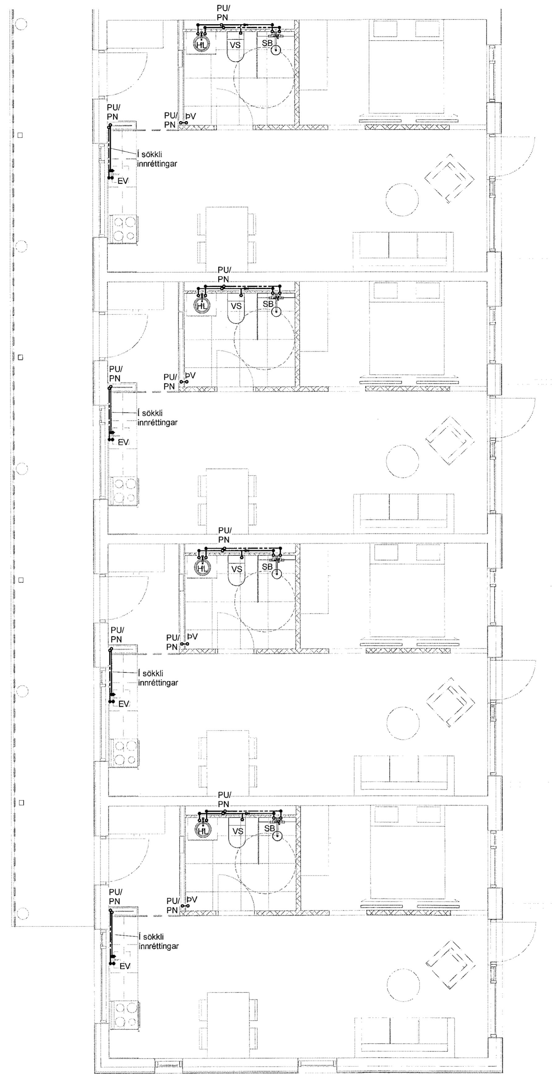
1 2. hæð - 4 1 : 50
