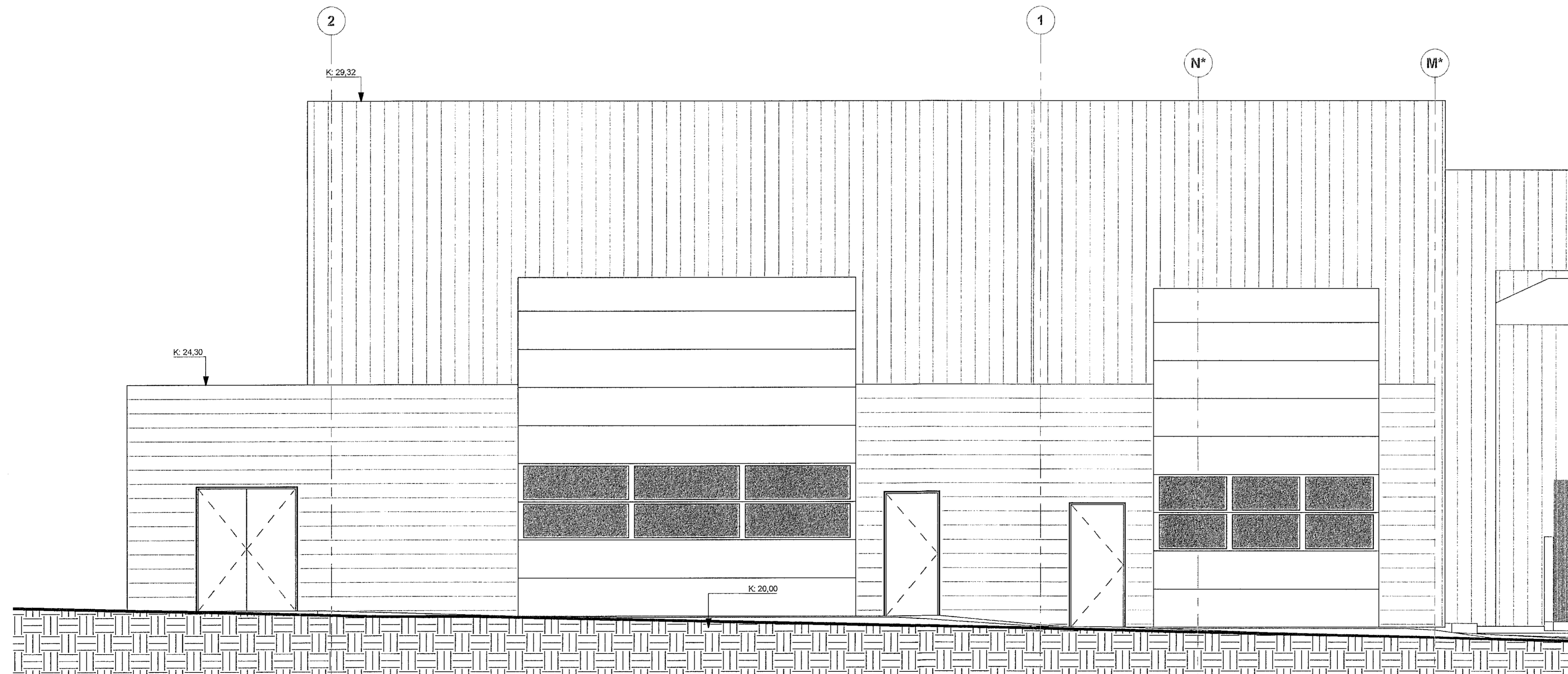
1 Austur 50 1:50
