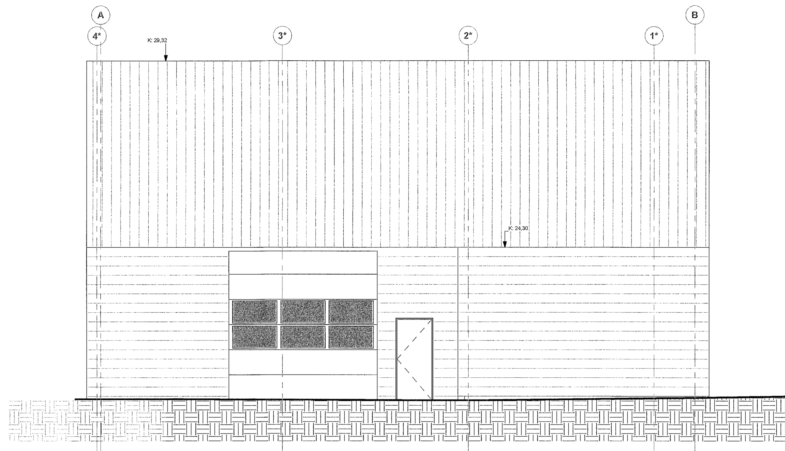
1 Austur 50 1:50
