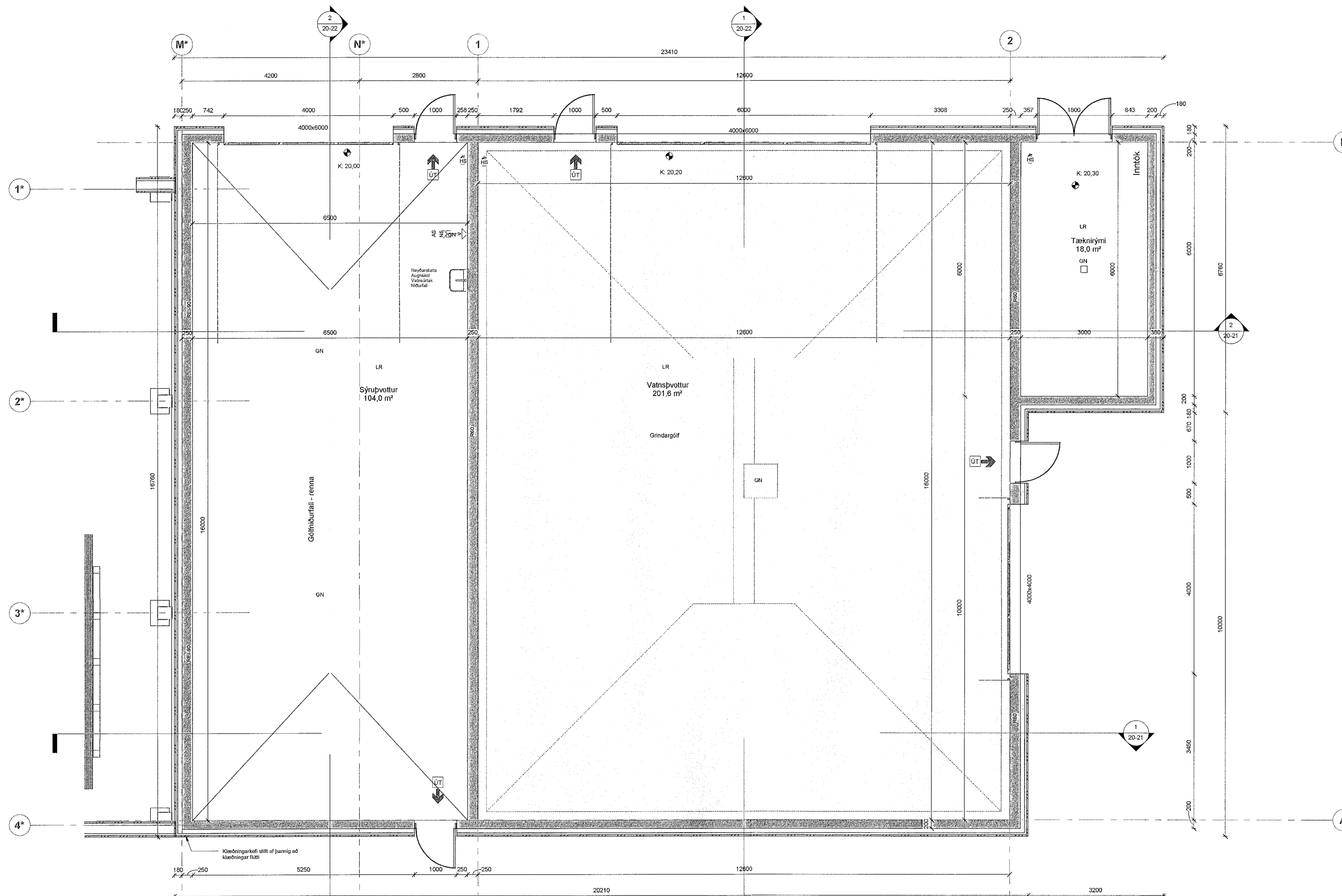
1. Hæð 50 1 : 50
