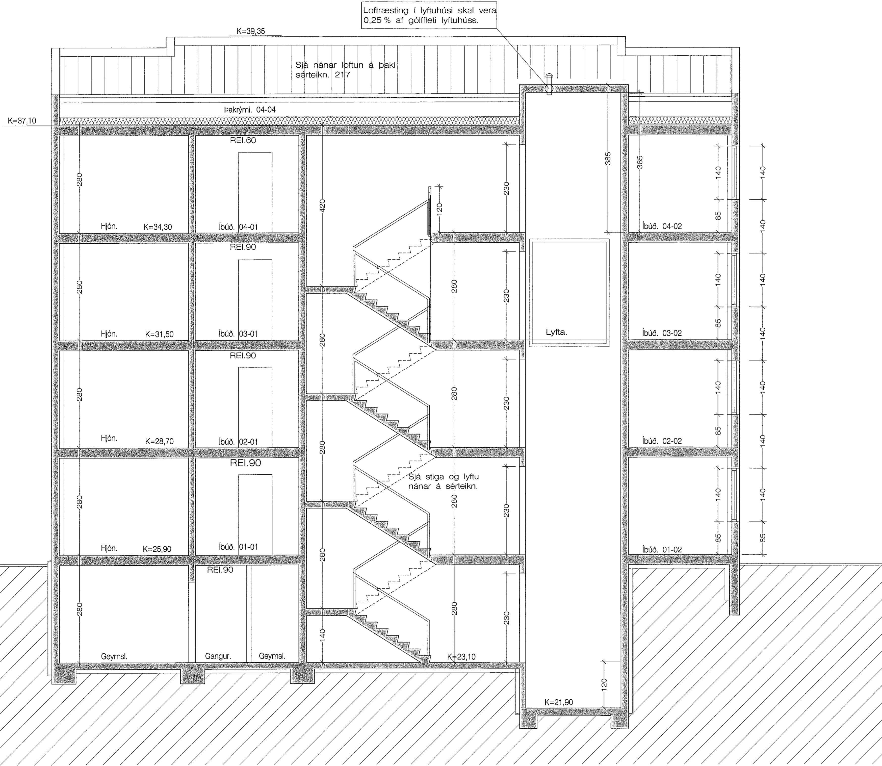
Sneiðing B - B 1 : 50
