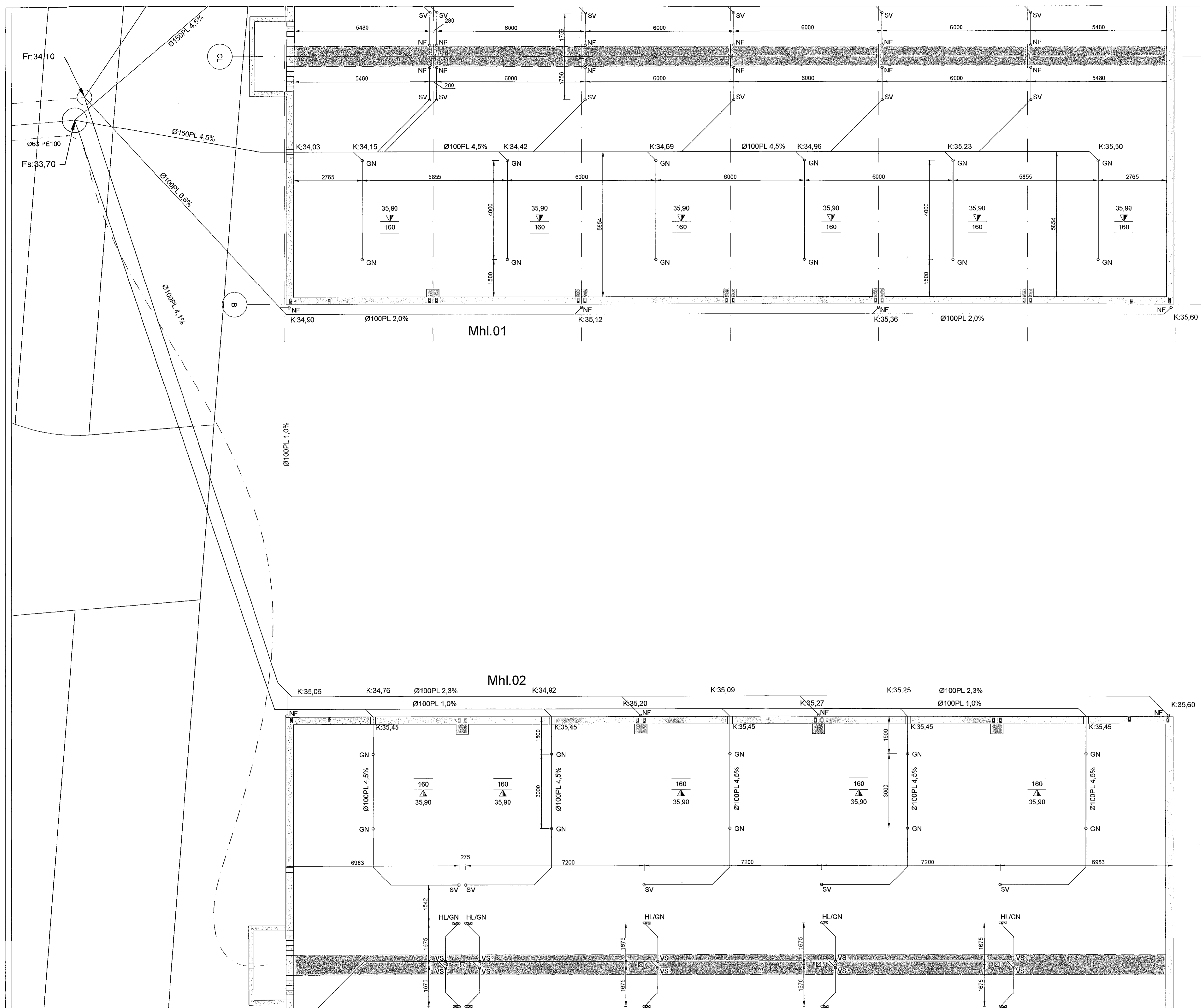
GRUNNMYND - FRÆRENNSLI 1:75 (A1)
