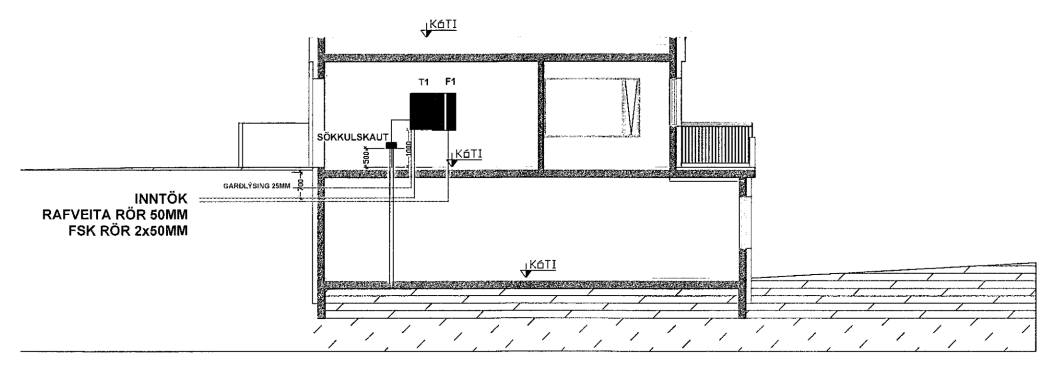
Sniðmynd 1:100
