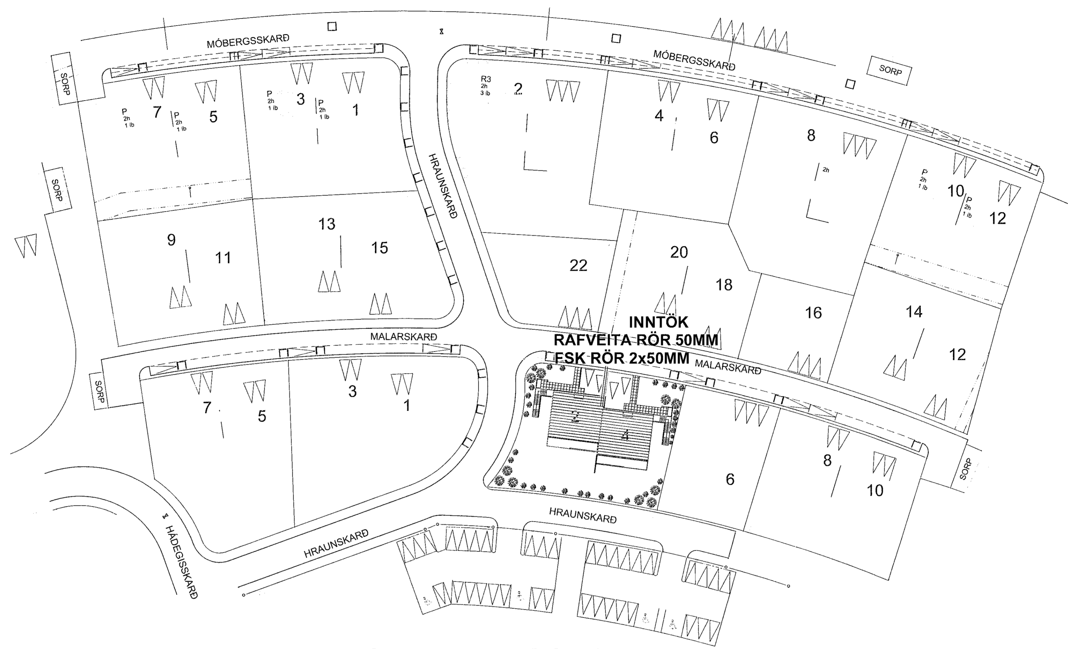
Afstöðumynd 1:500
