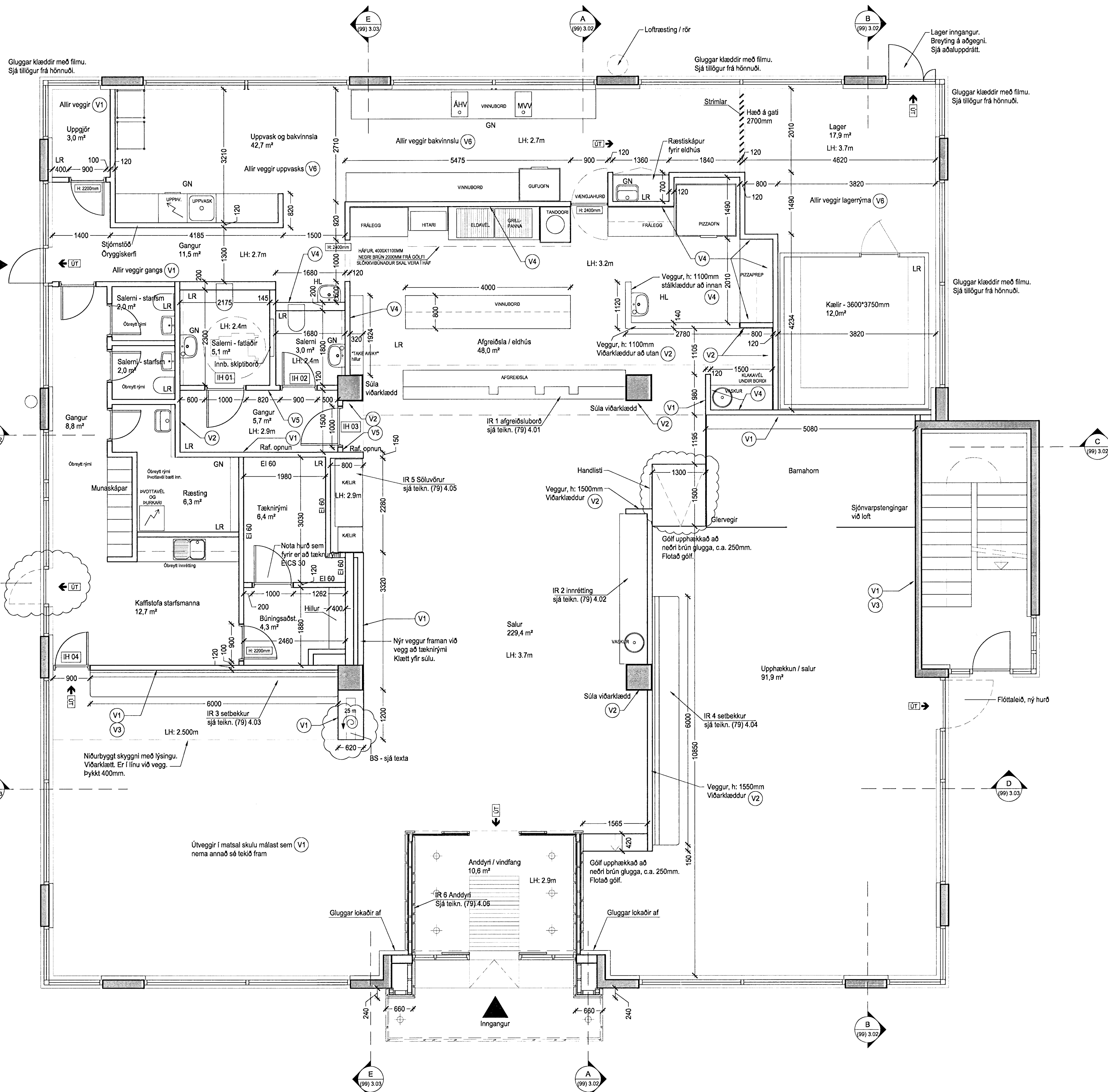
1 GRUNNMÝND 1.HÆÐ 1:50
