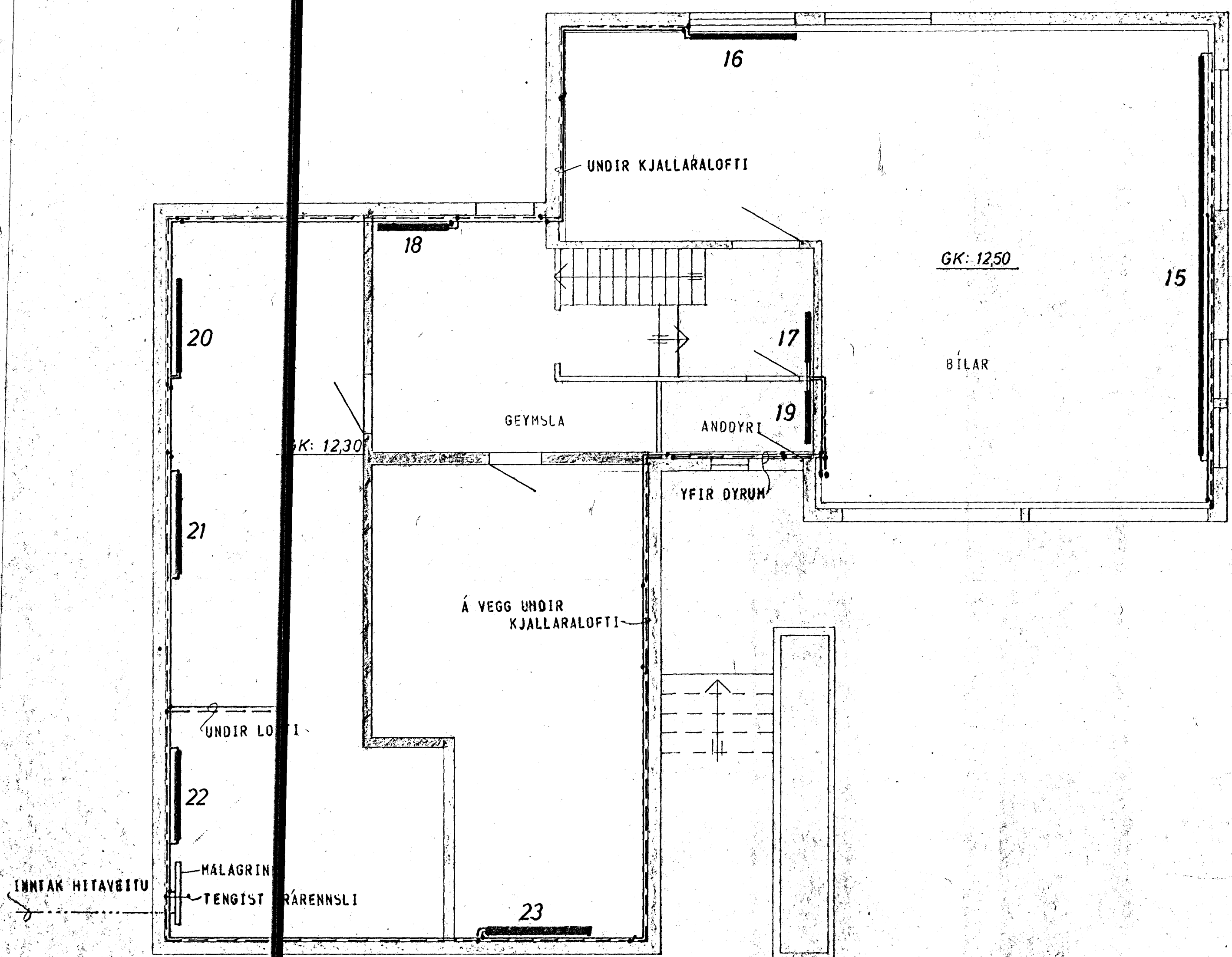
GRUNNMYND KJALLARA 1:50
