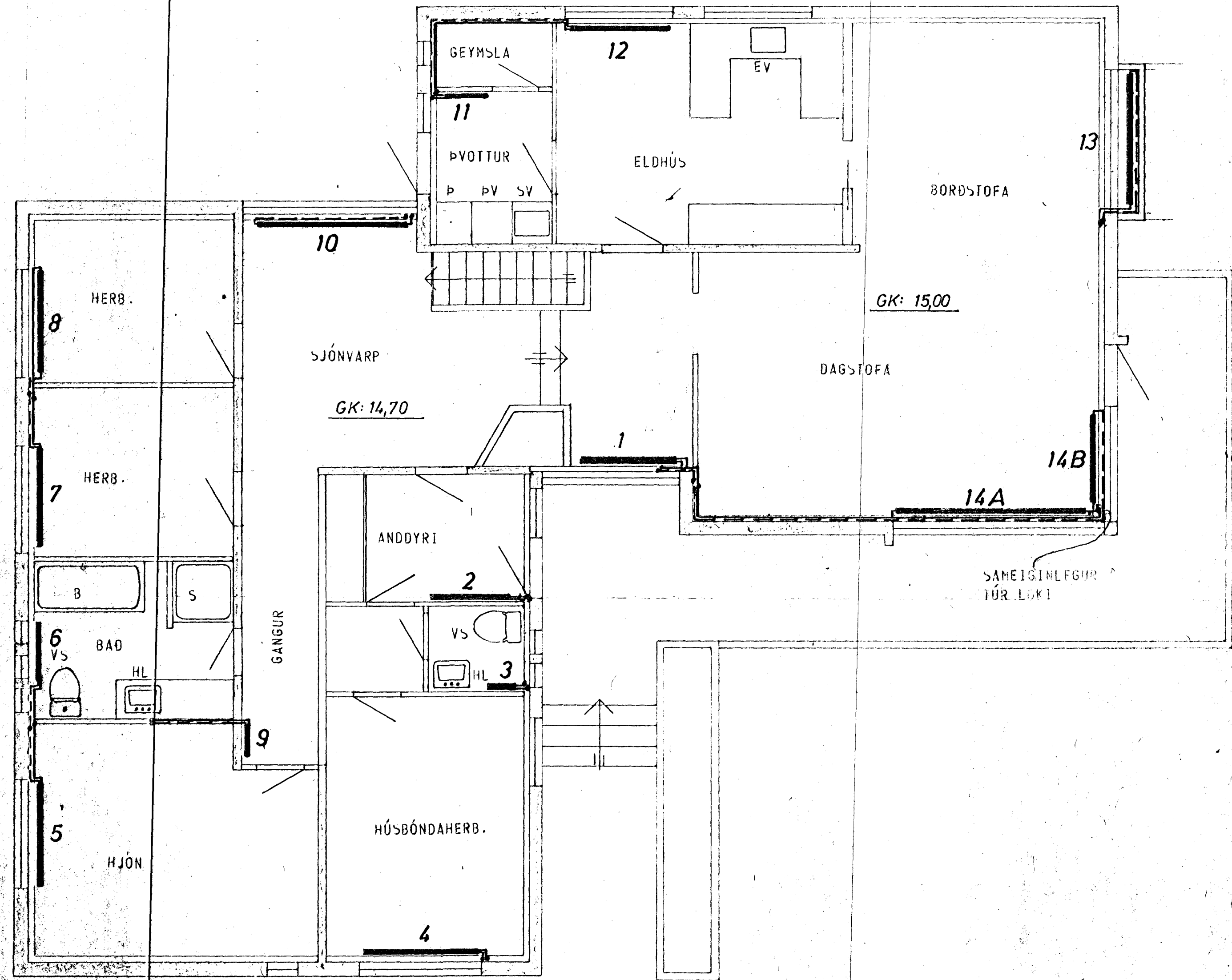
GRUNNMYND HÆÐAR 1:50
