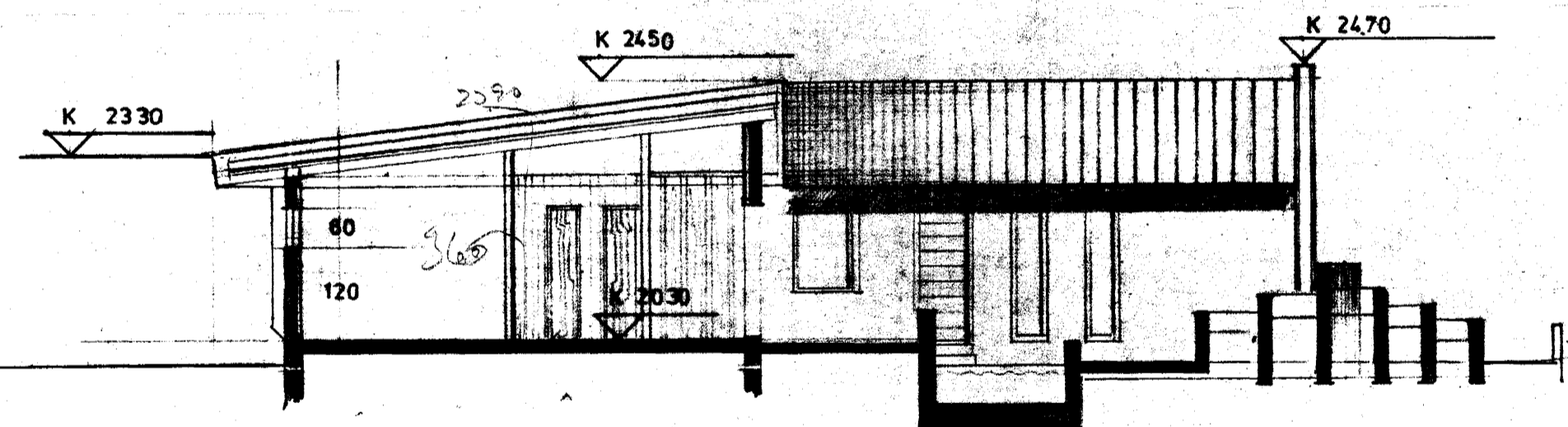
SNID A-A
