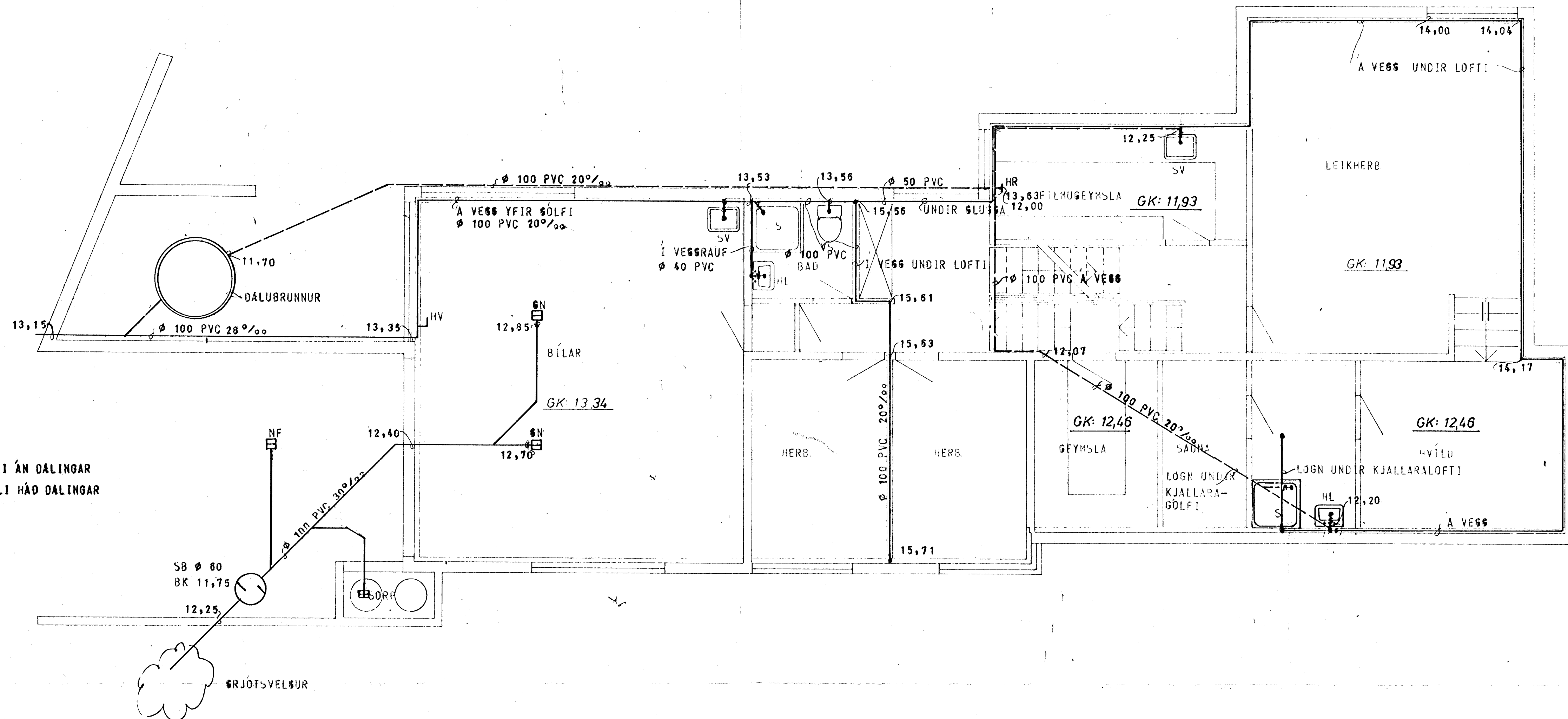
GRUNNMYND NEDRI HÆÐAR 1:50
