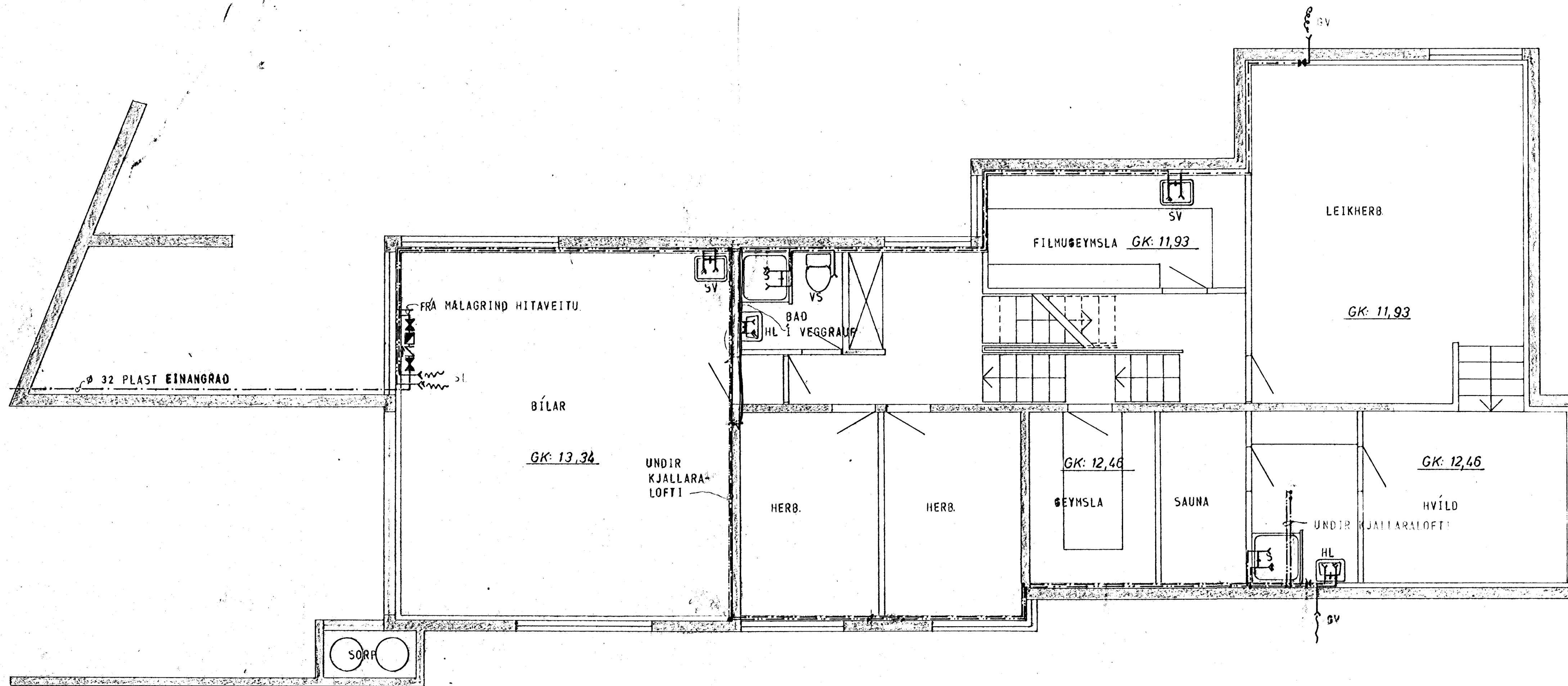
GRUNNMYND NEDRI HÆÐAR 1:50
