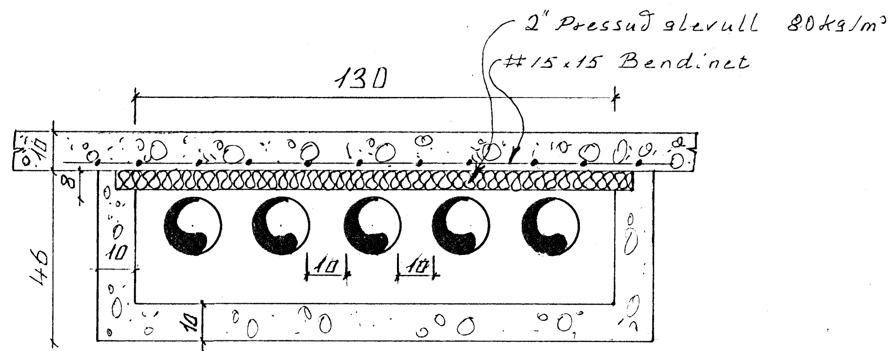
Snið B-B 1:10
