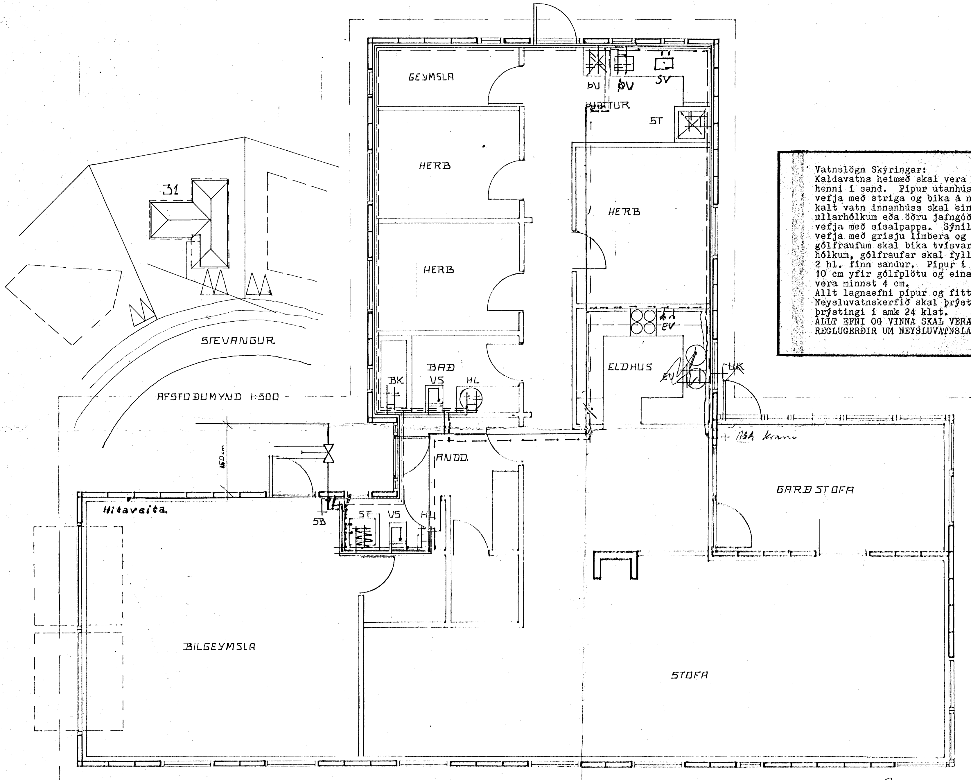
GRUNNMYND 1:50
