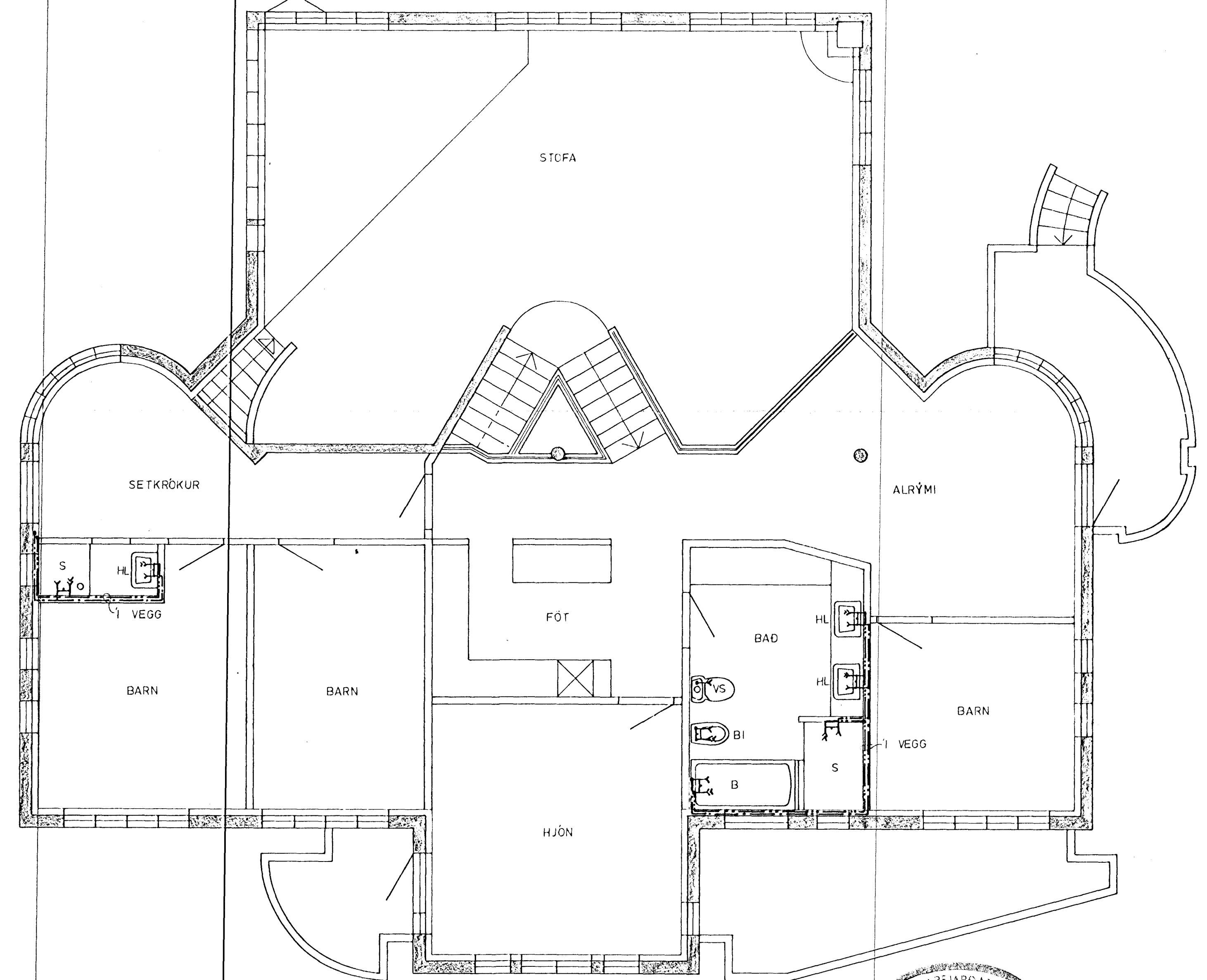
GRUNNMYND EFR HÆÐ 1 : 50
