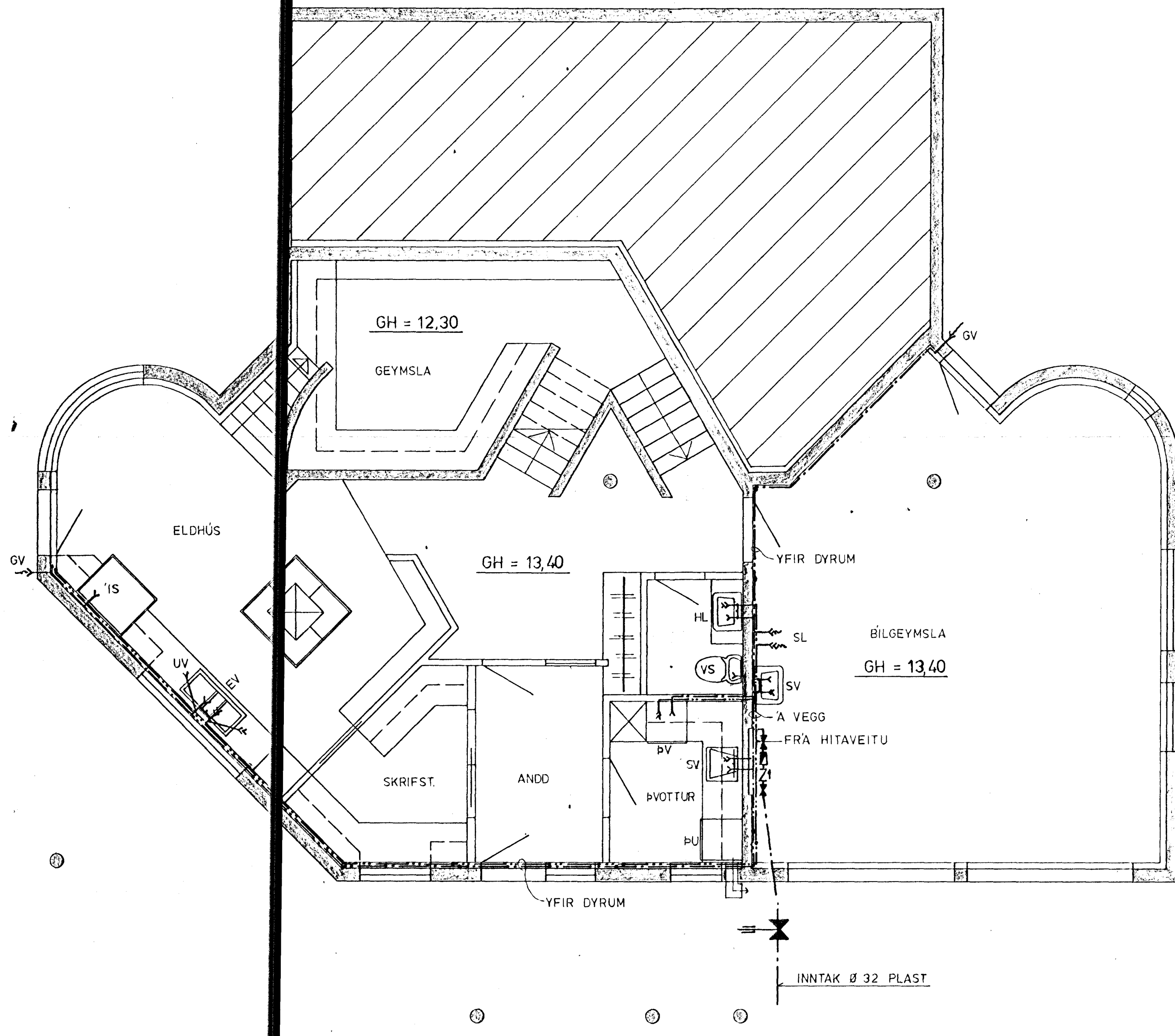
GRUNNMYND NEDRI HÆÐ 1 : 50
