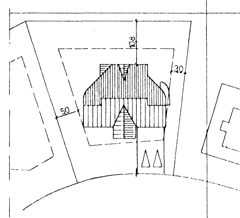
AFSTADA 1:500
