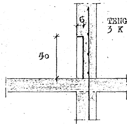
SNID - B 1:20
