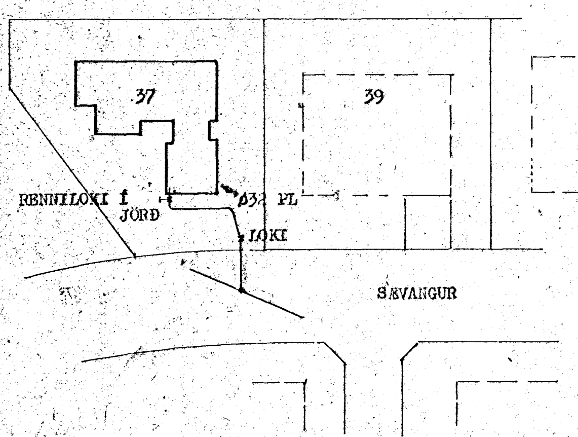
AFSTÖÐUMYND 1:500
