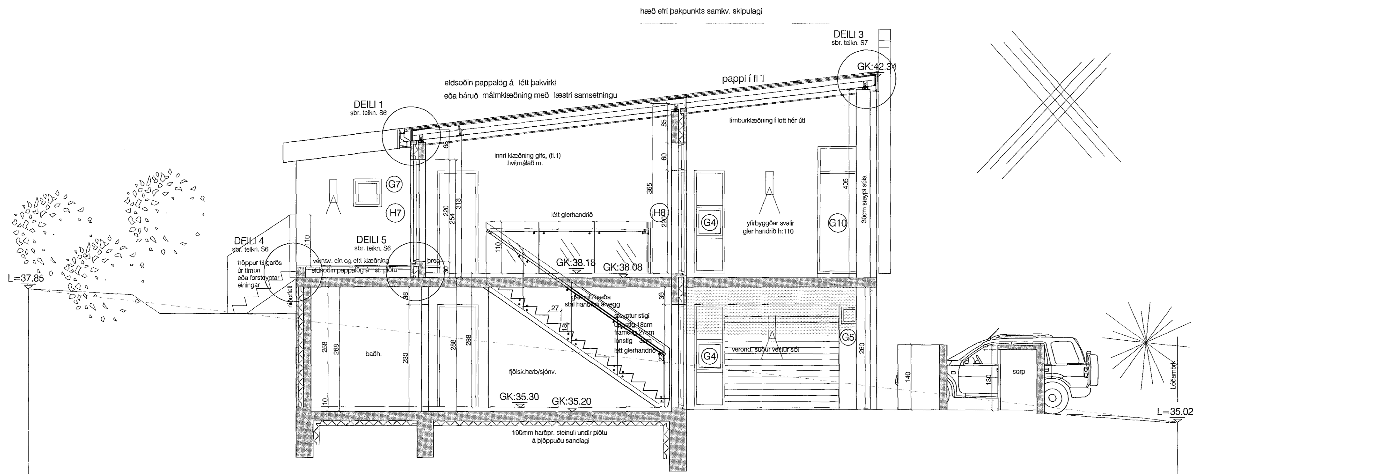
sneiðing B-B
