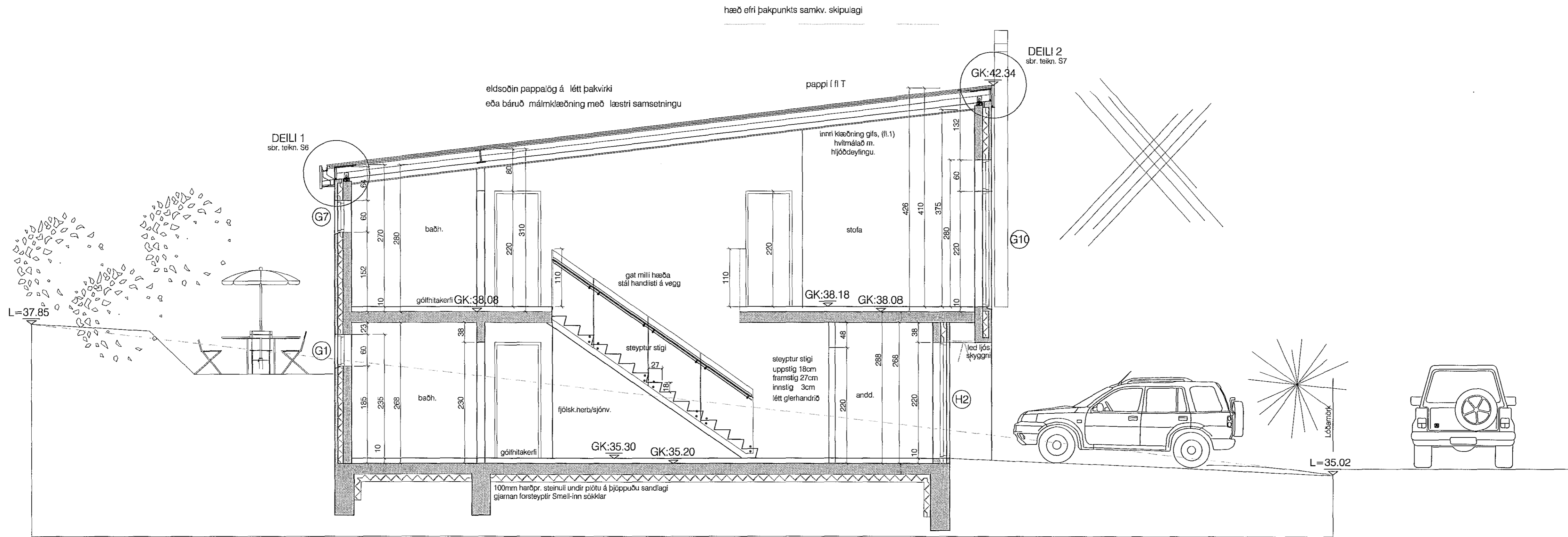
sneiðing A-A
