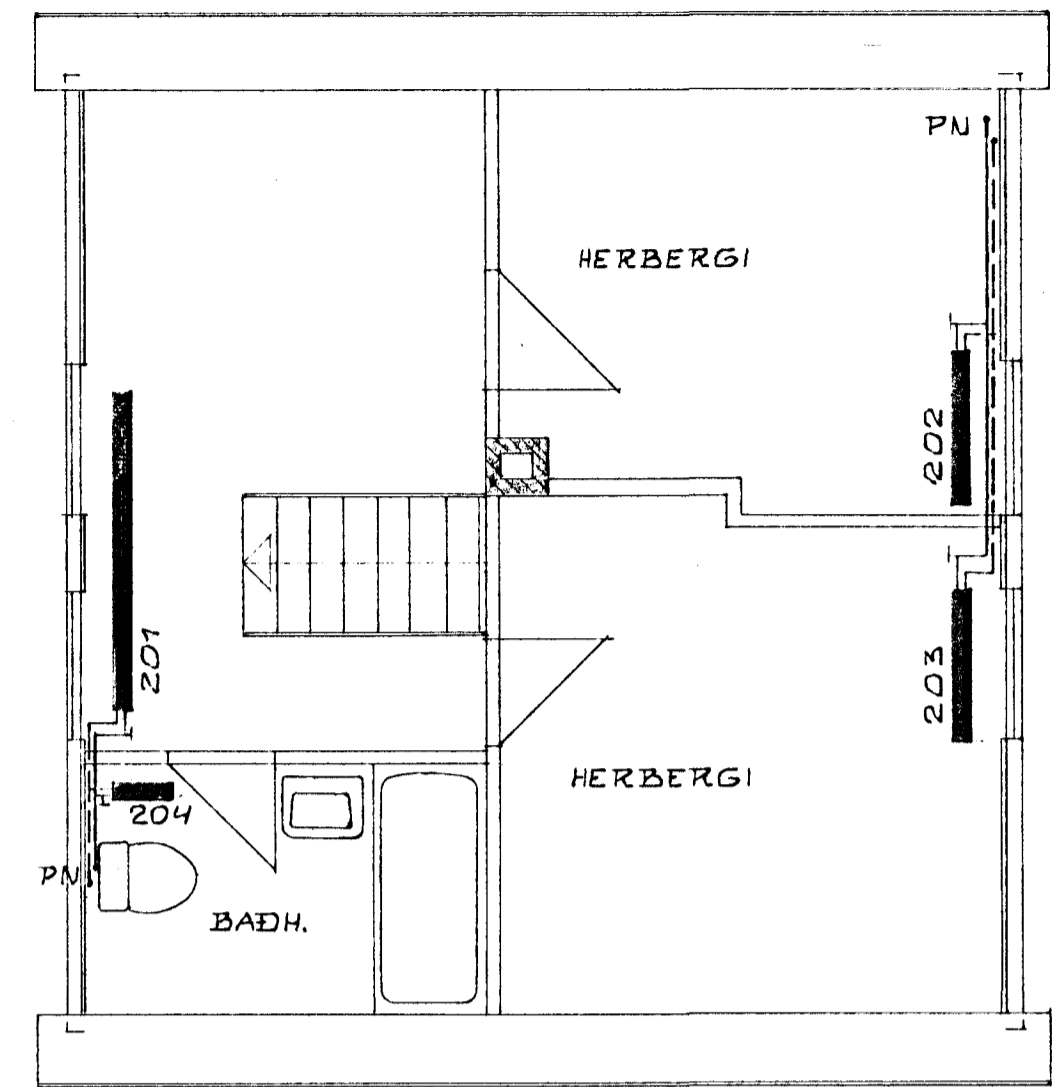
RISHÆÐ 1:50
