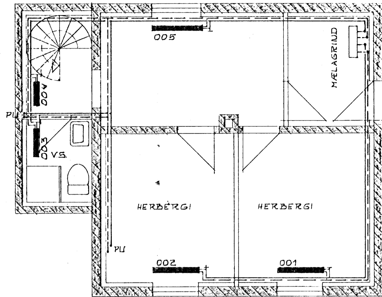
KJALLARI 1:50
