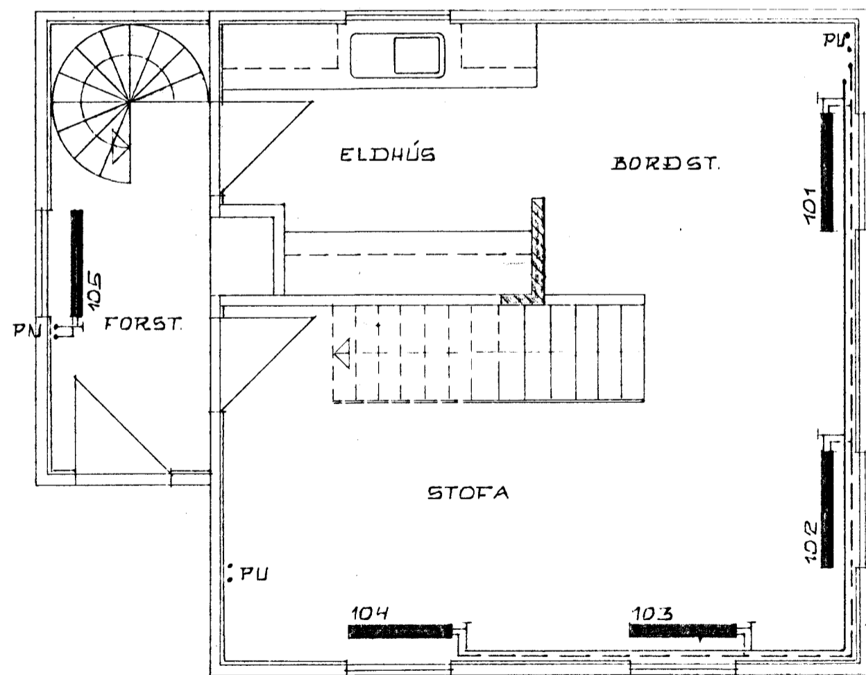
1. HÆÐ 1:50
