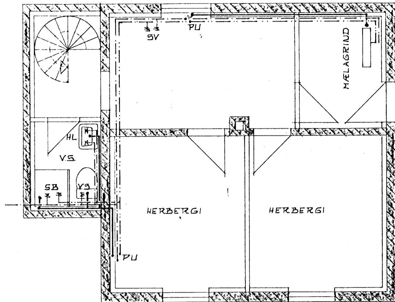
KJALLARI 1:50
