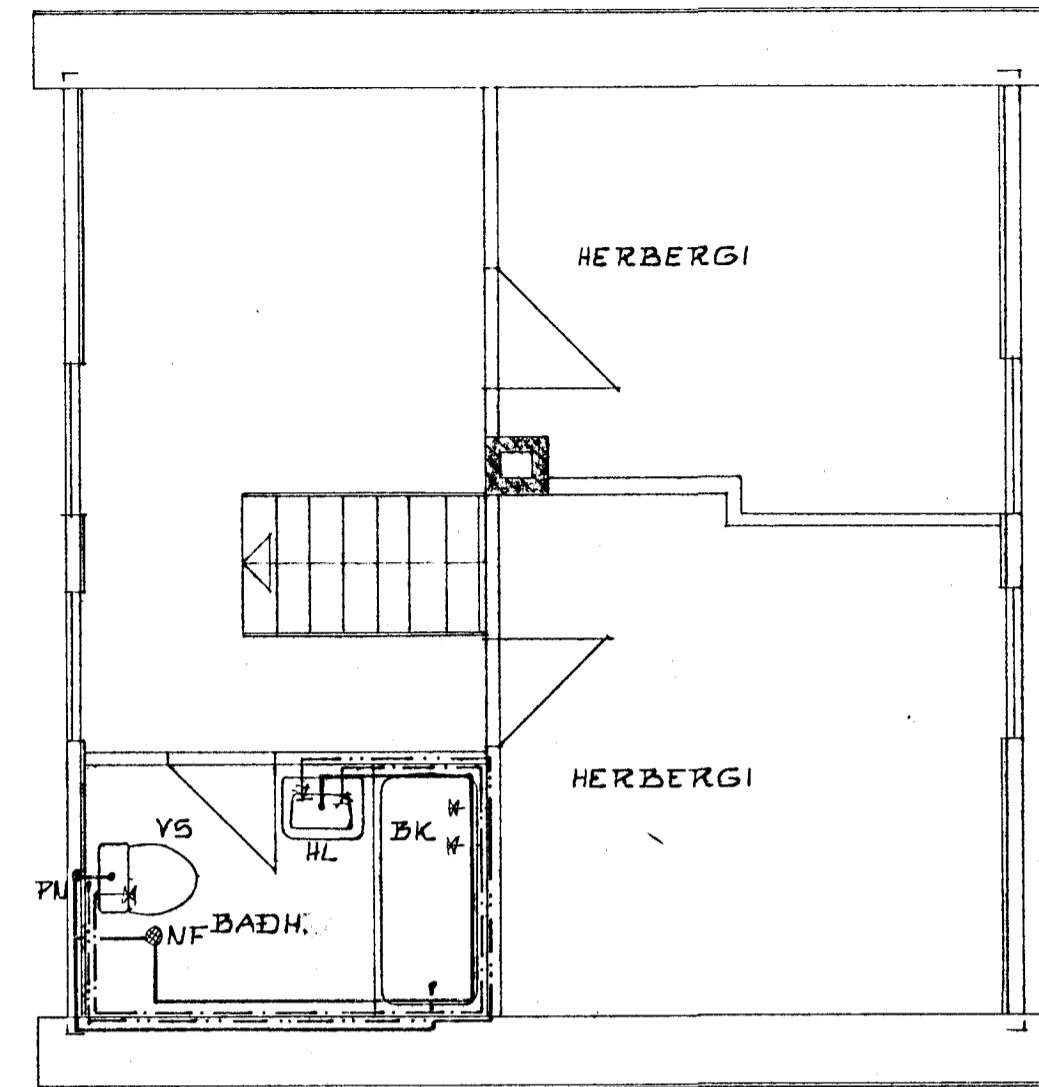
RISHÆÐ 1:50
