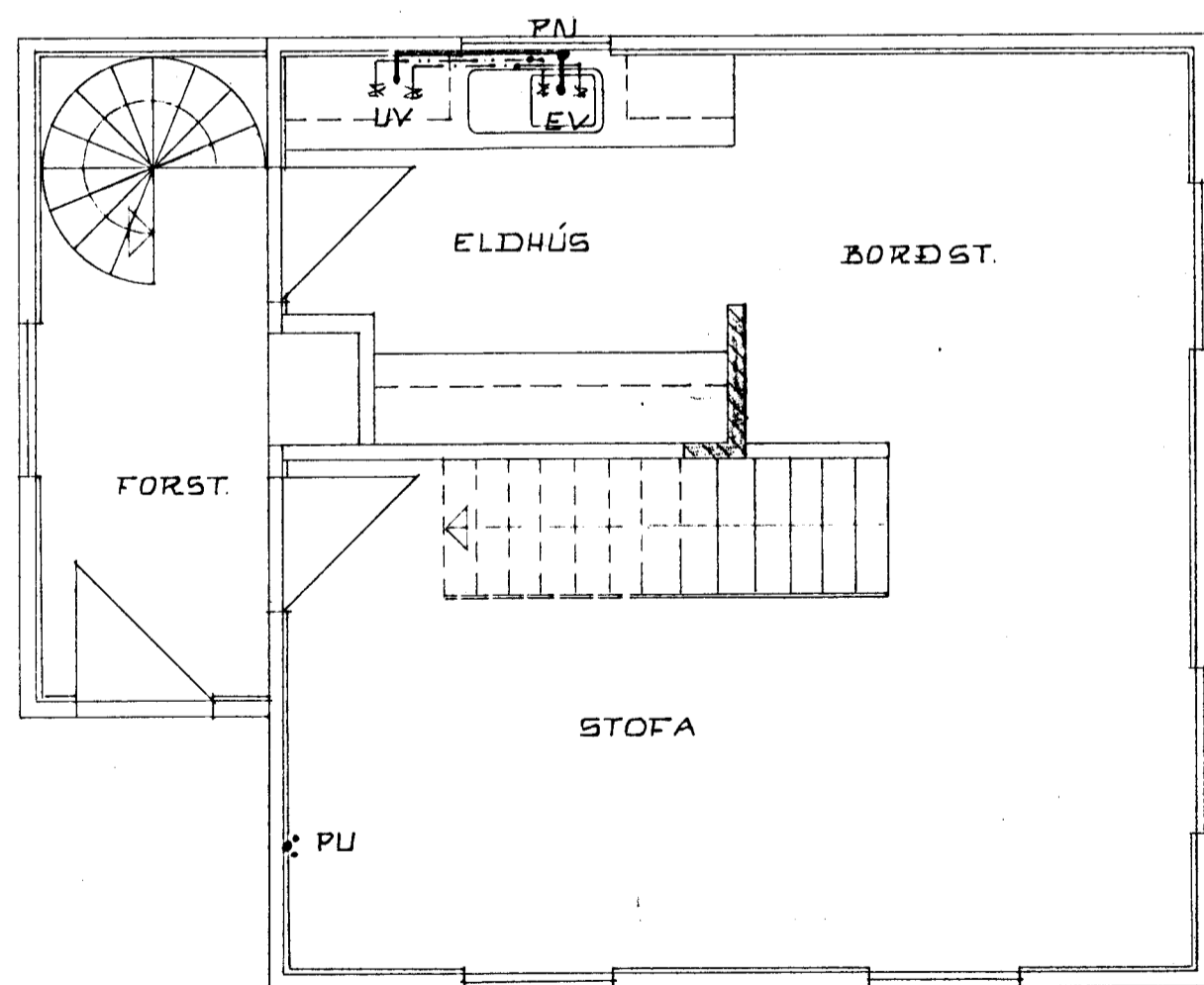
1. HÆÐ 1:50
