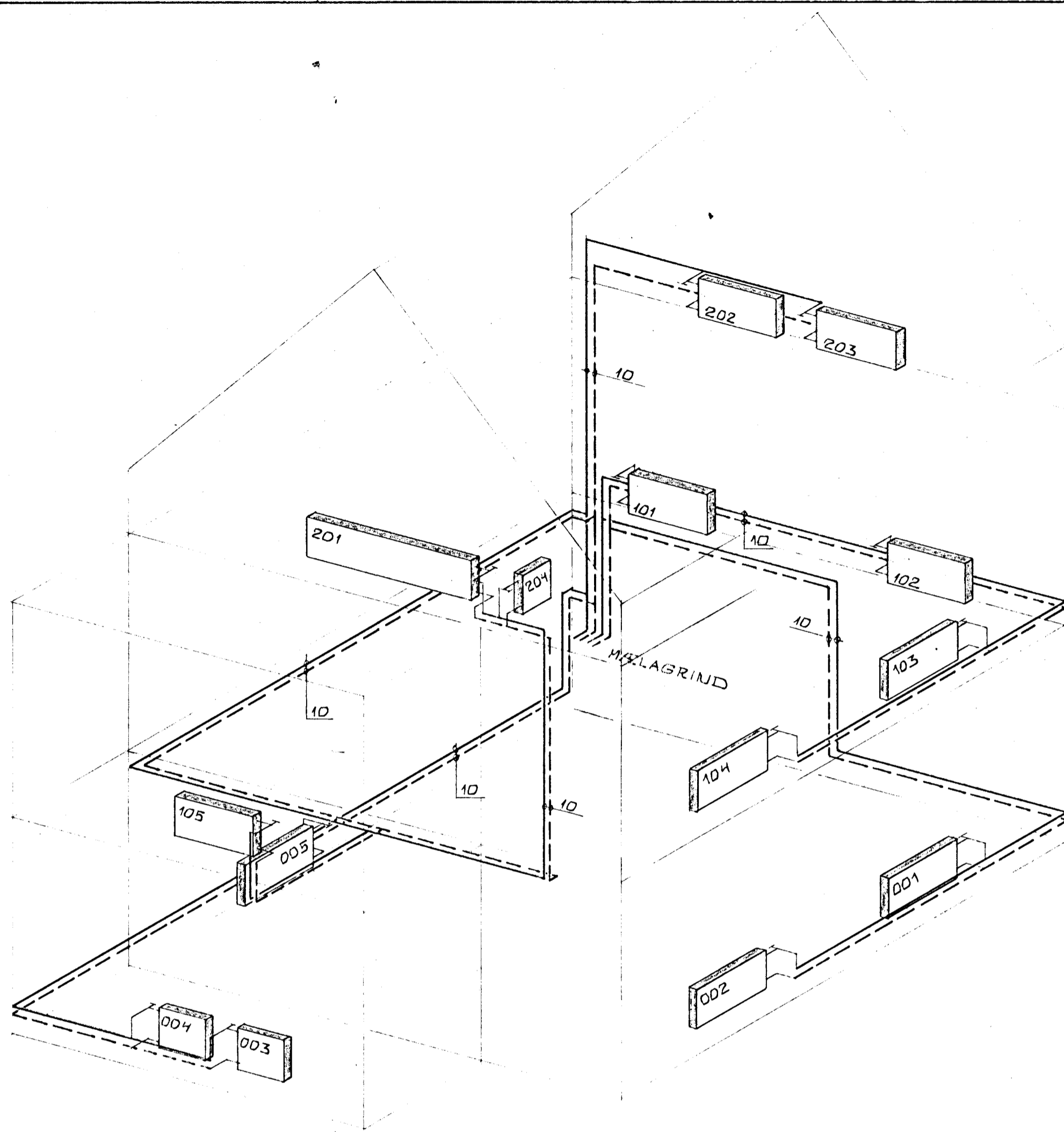
RÚMMYND HITALAGNA 1:50
