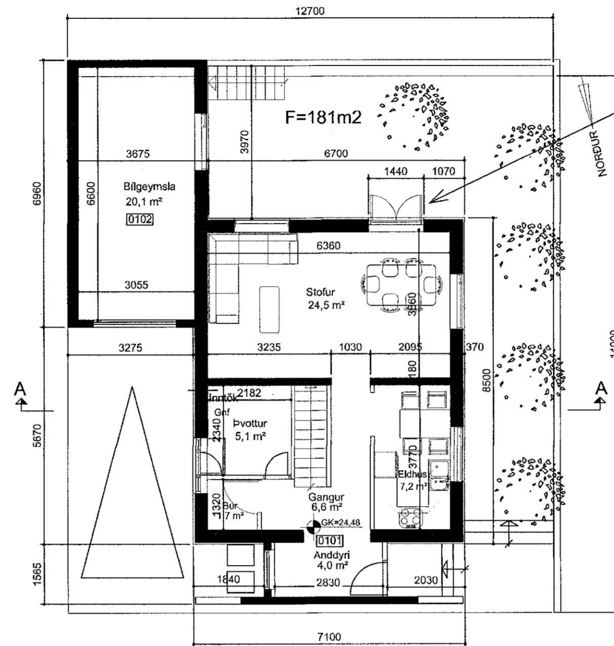
GRUNNMYND NEDRI HÆÐ, 1:100
