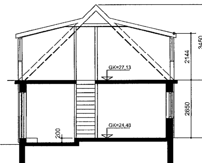
SKURÐUR A, 1:100
