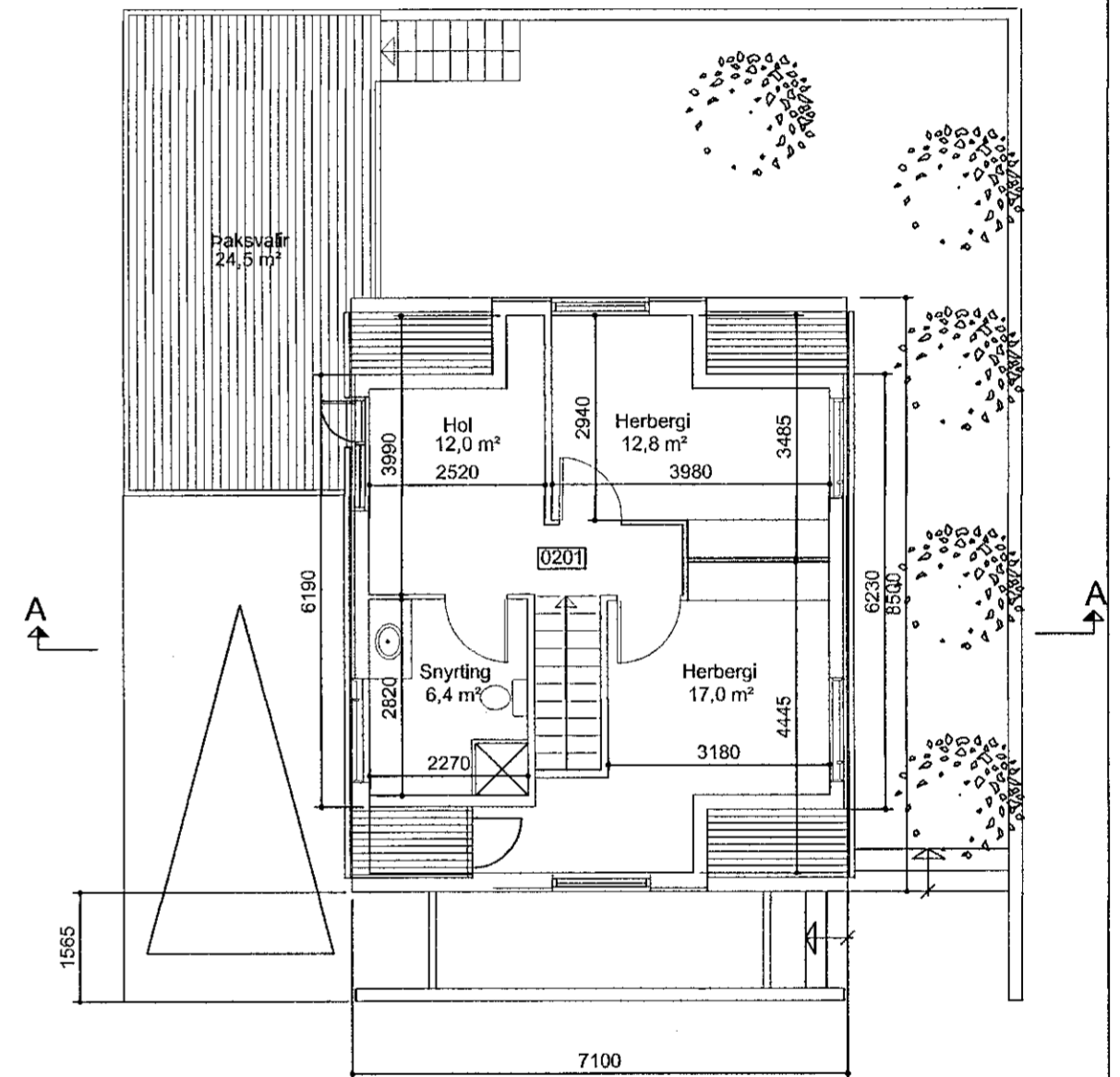
GRUNNMYND RISHÆÐ, 1:100
