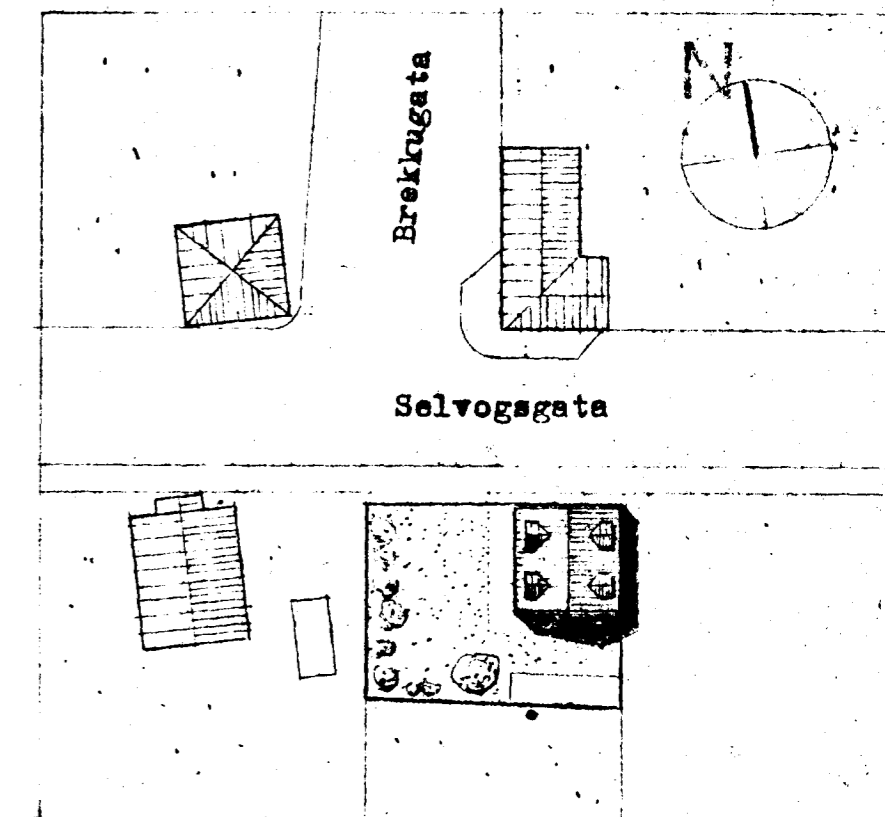
afstöðumynd 1 : 500
