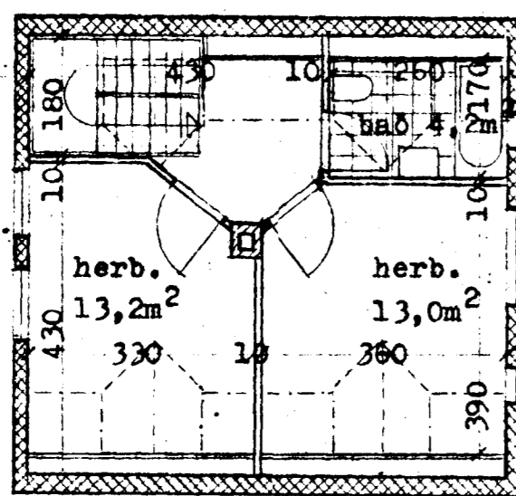
grunnmynd rishæðar
