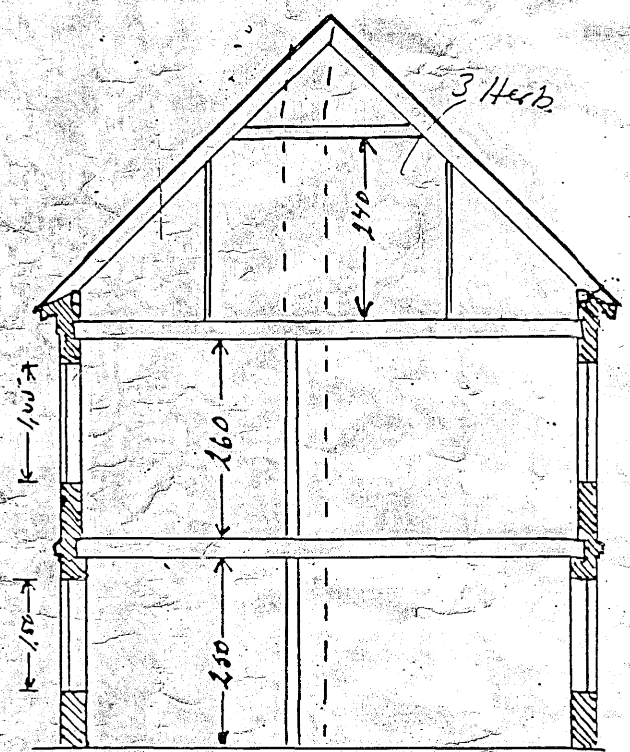
Skurður A-A
