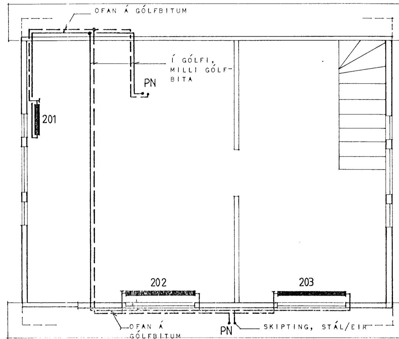
RISHÆÐ mkv. 1:50
