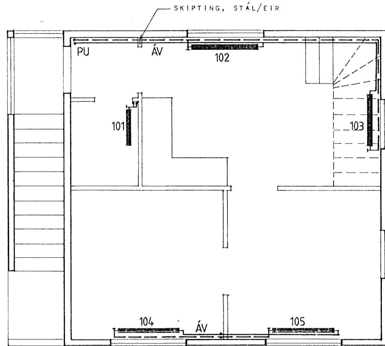
MIDHÆÐ mkv. 1:50
