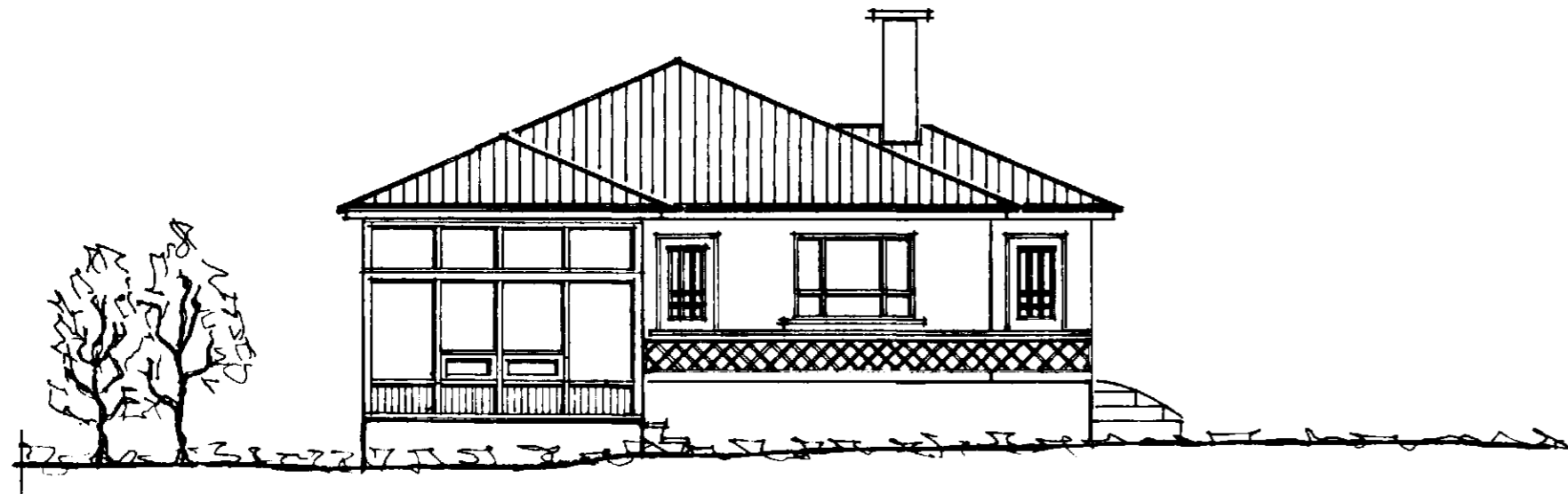
SUDVESTUR M.1:100
