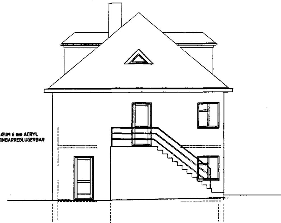
VESTURHLIÐ 1:100
