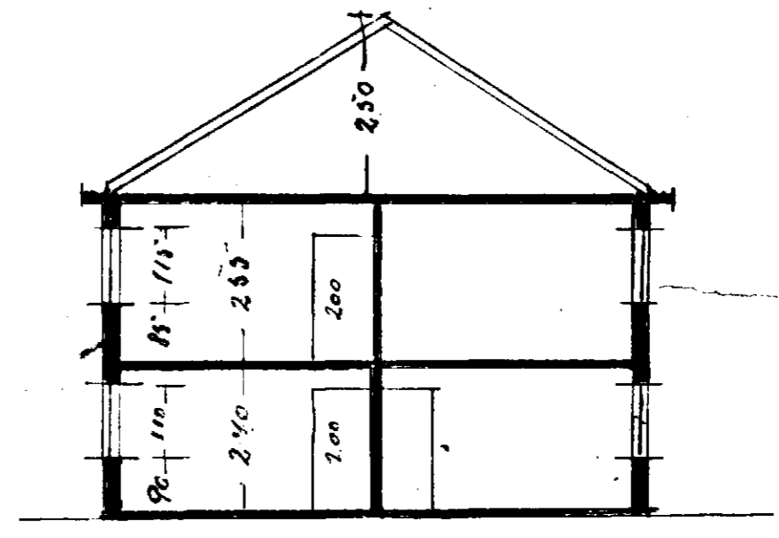
Skurðarsn. A-B
