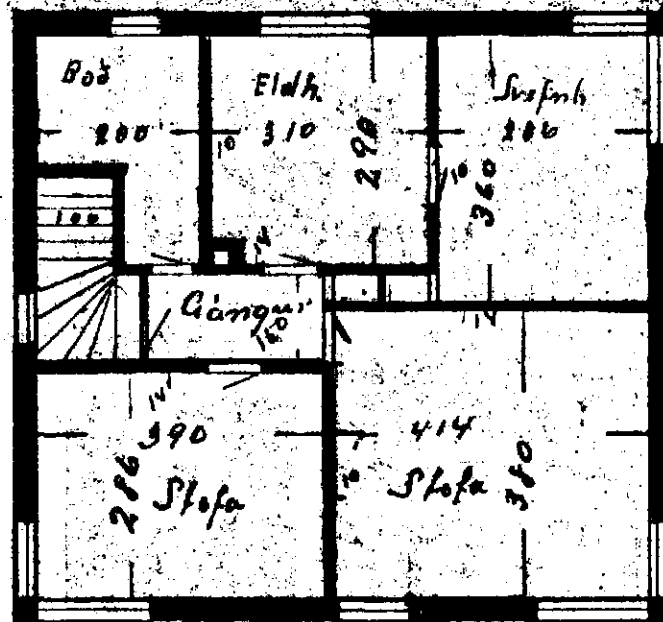
1. Hæð.
