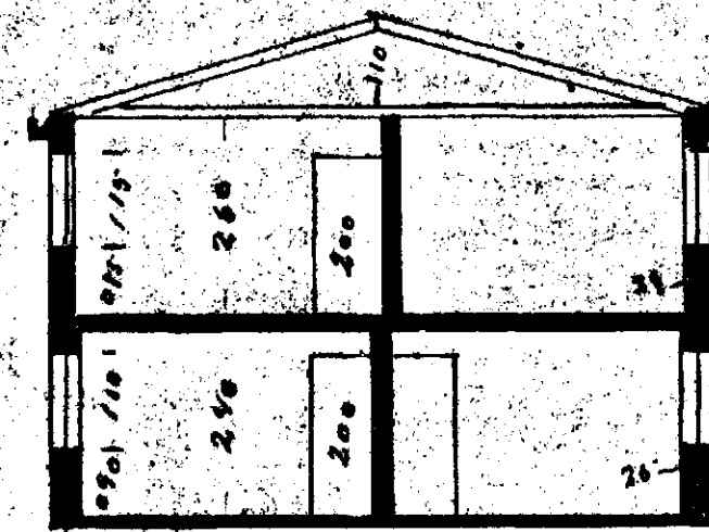
SKURÐUR A-B
