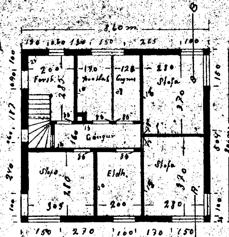
Kjallarahæð
