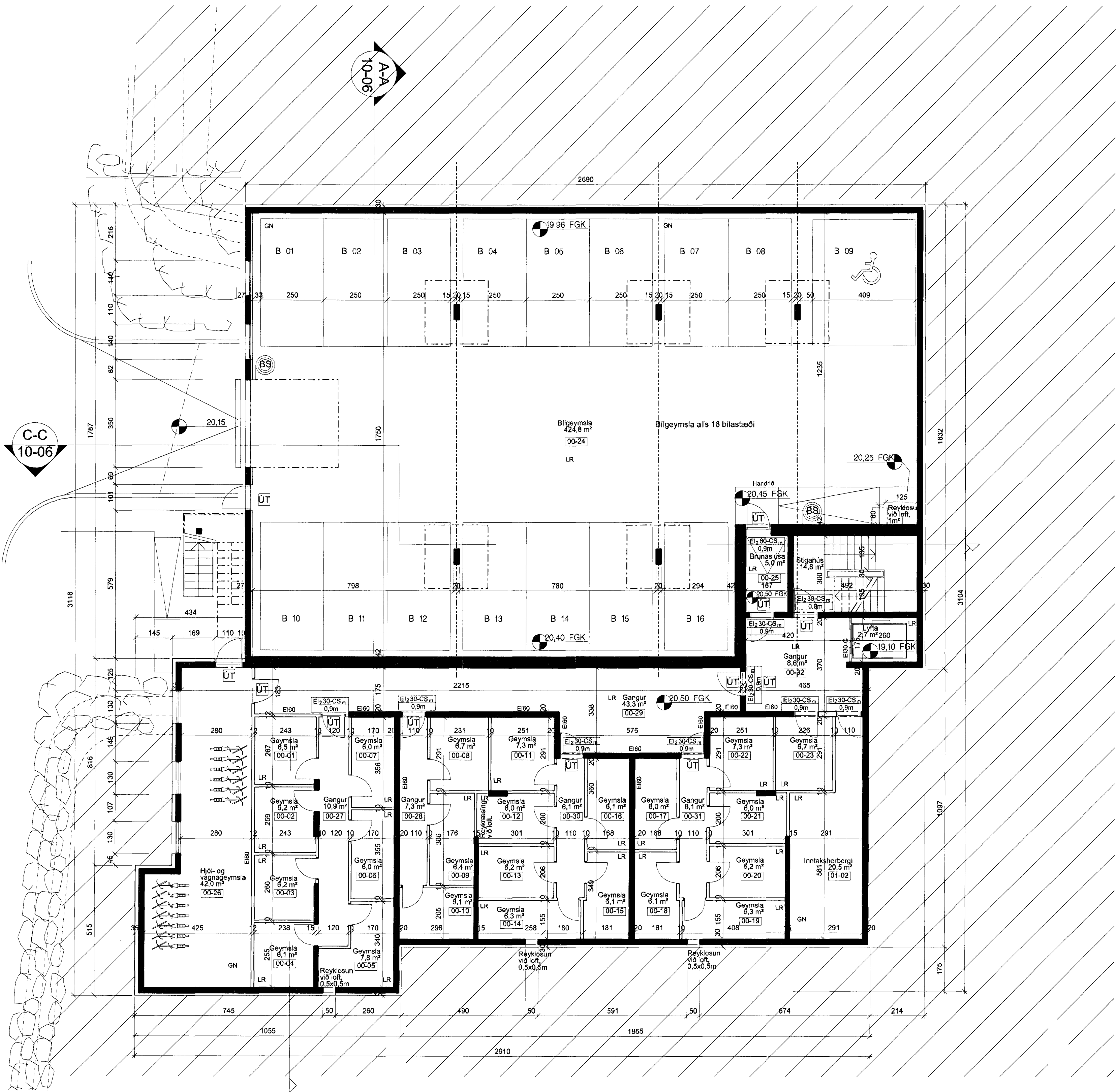
GRUNNMYND 1:100 KJALLARI
