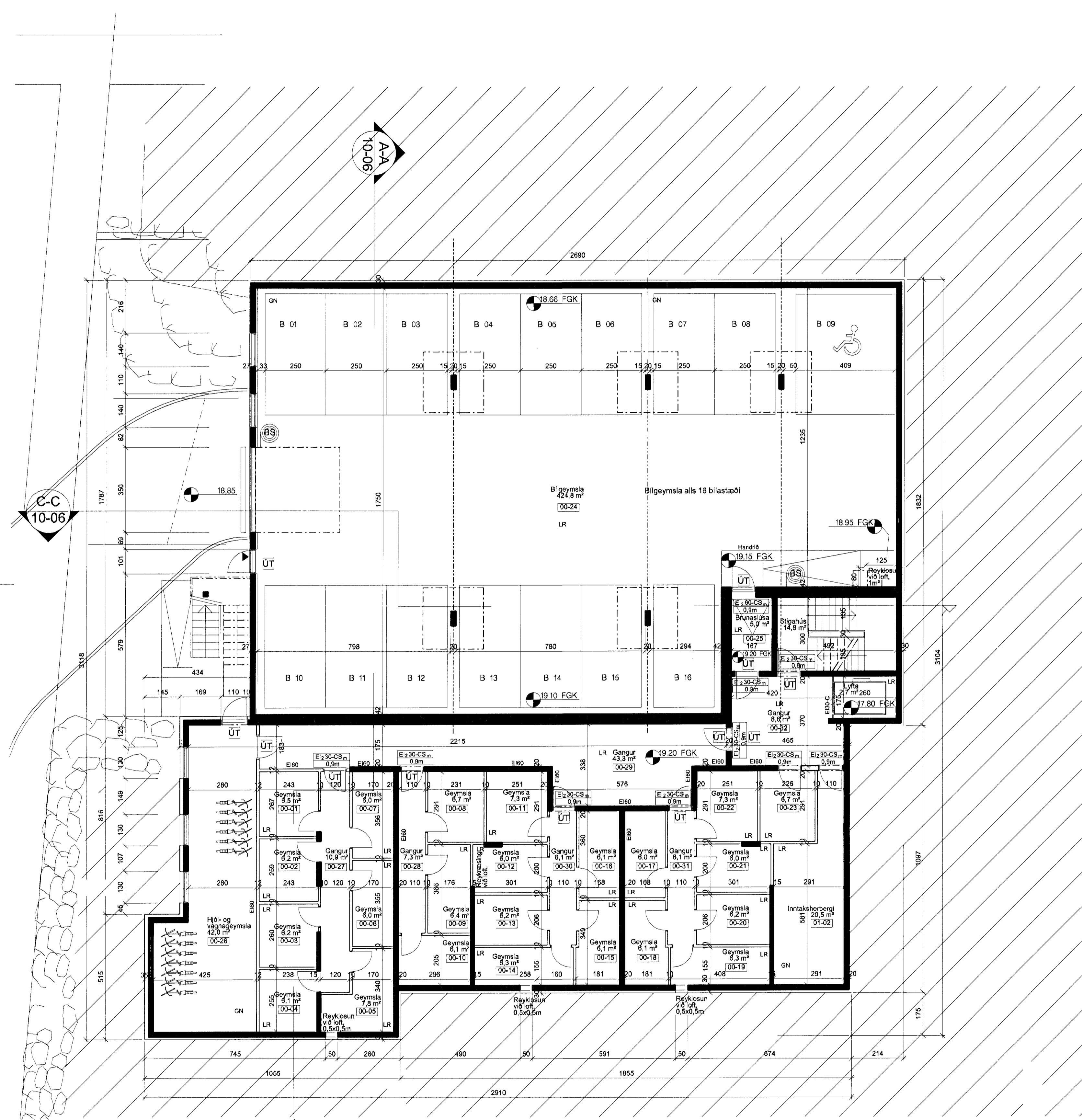
GRUNNMYND 1:100 KJALLARI
