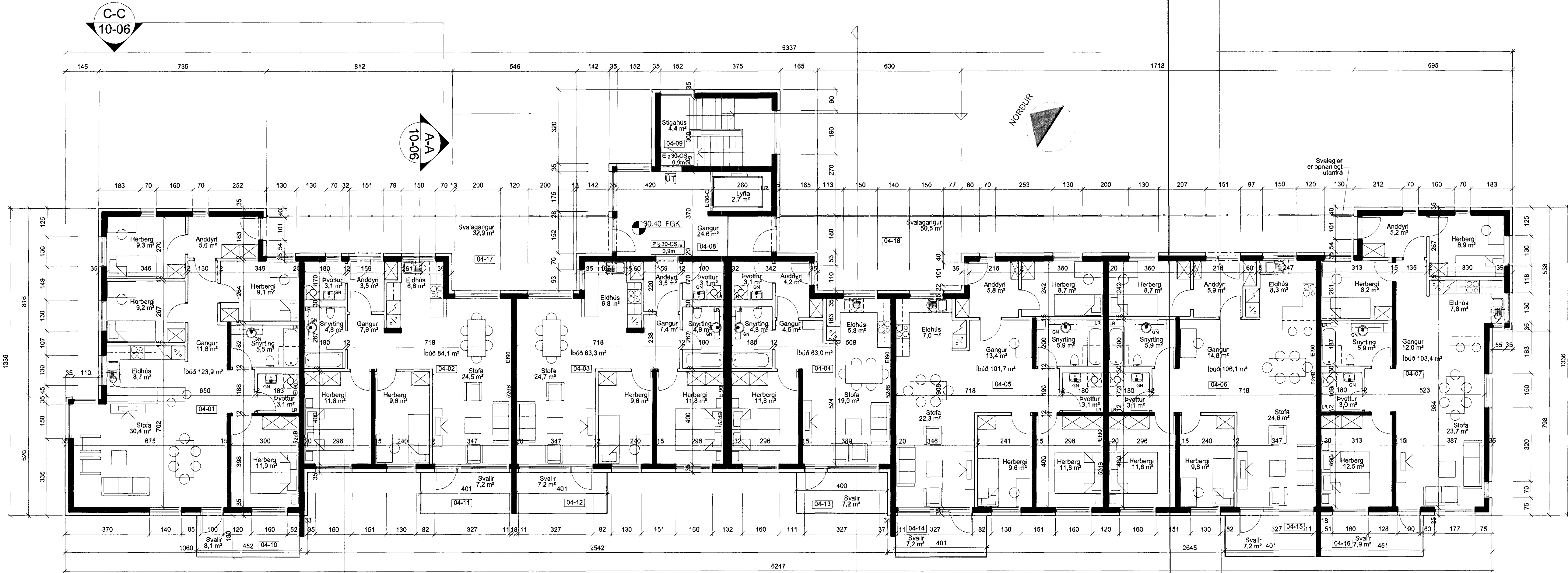
GRUNNMYND 1:100 4. HÆÐ
