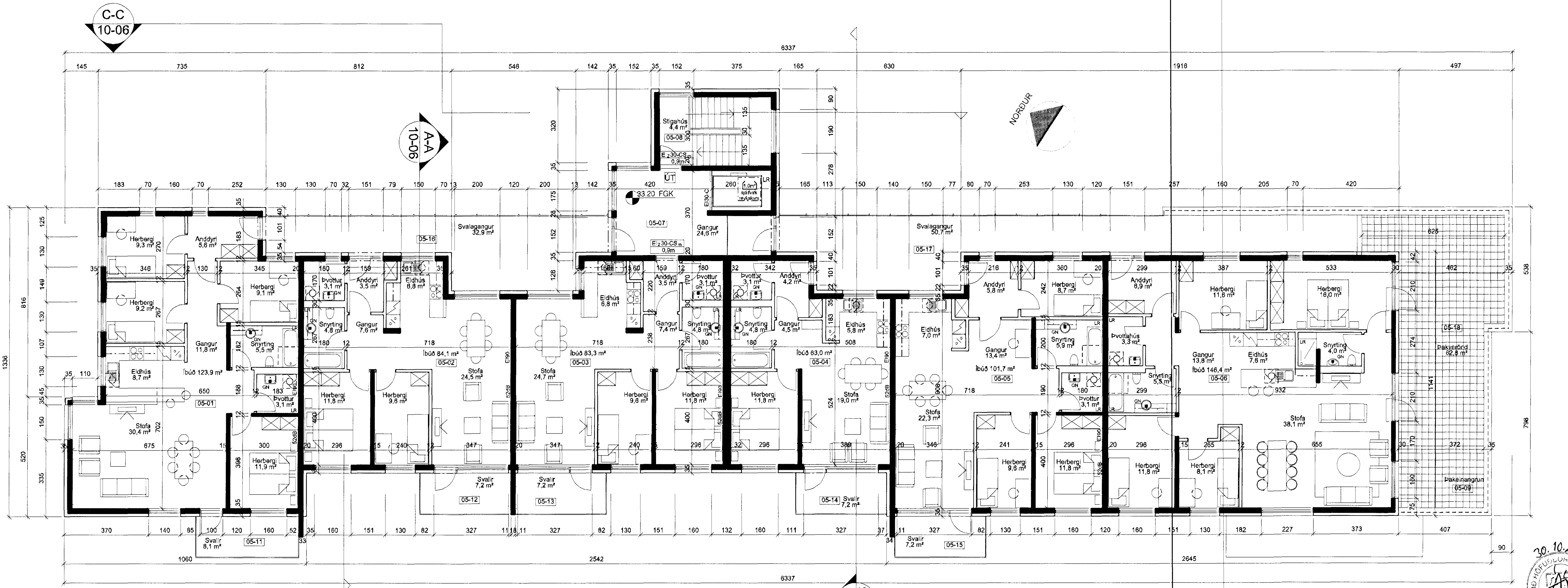
GRUNNMYND 1:100 5. HÆÐ
