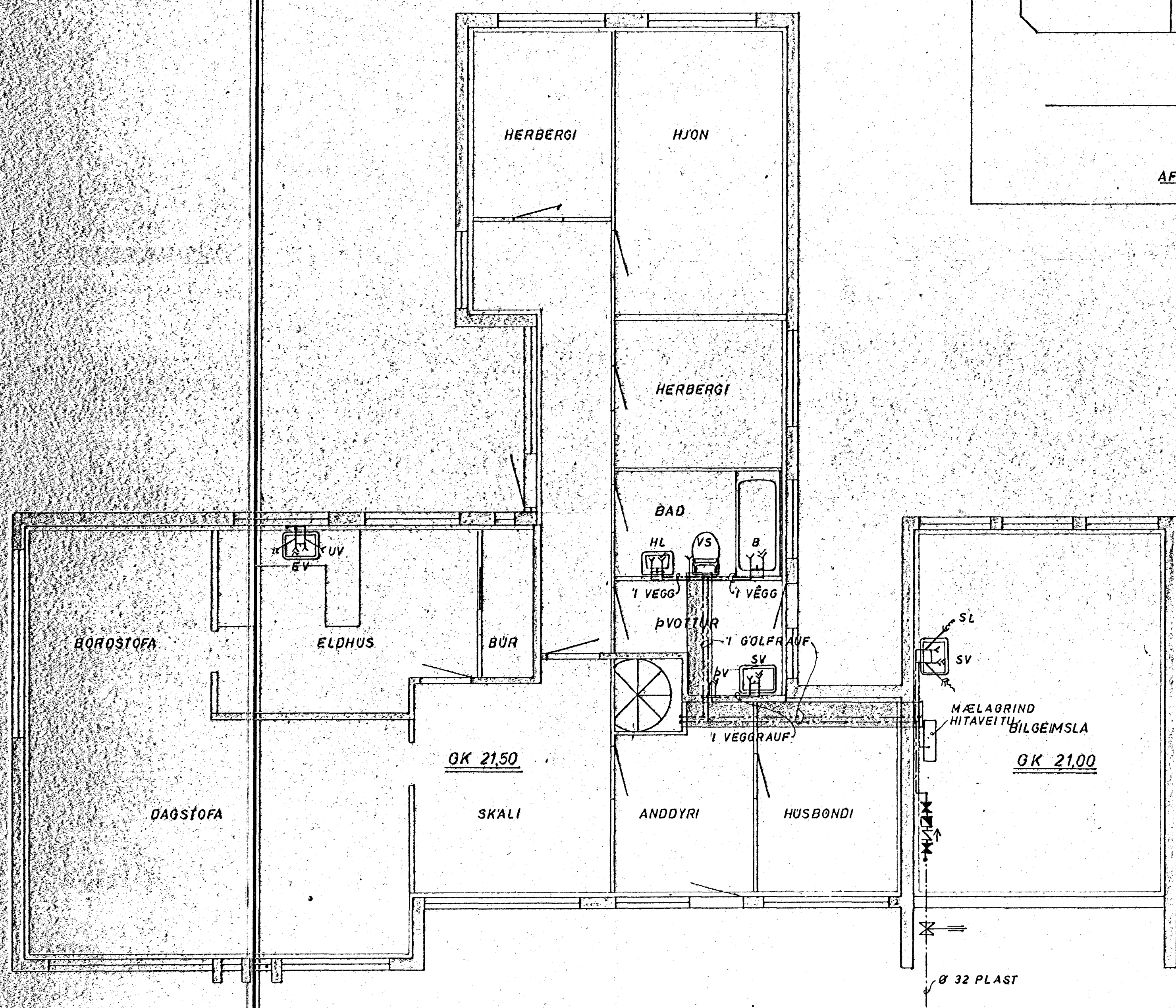
GRUNNMYND HÆÐAR MKV. 1:50
