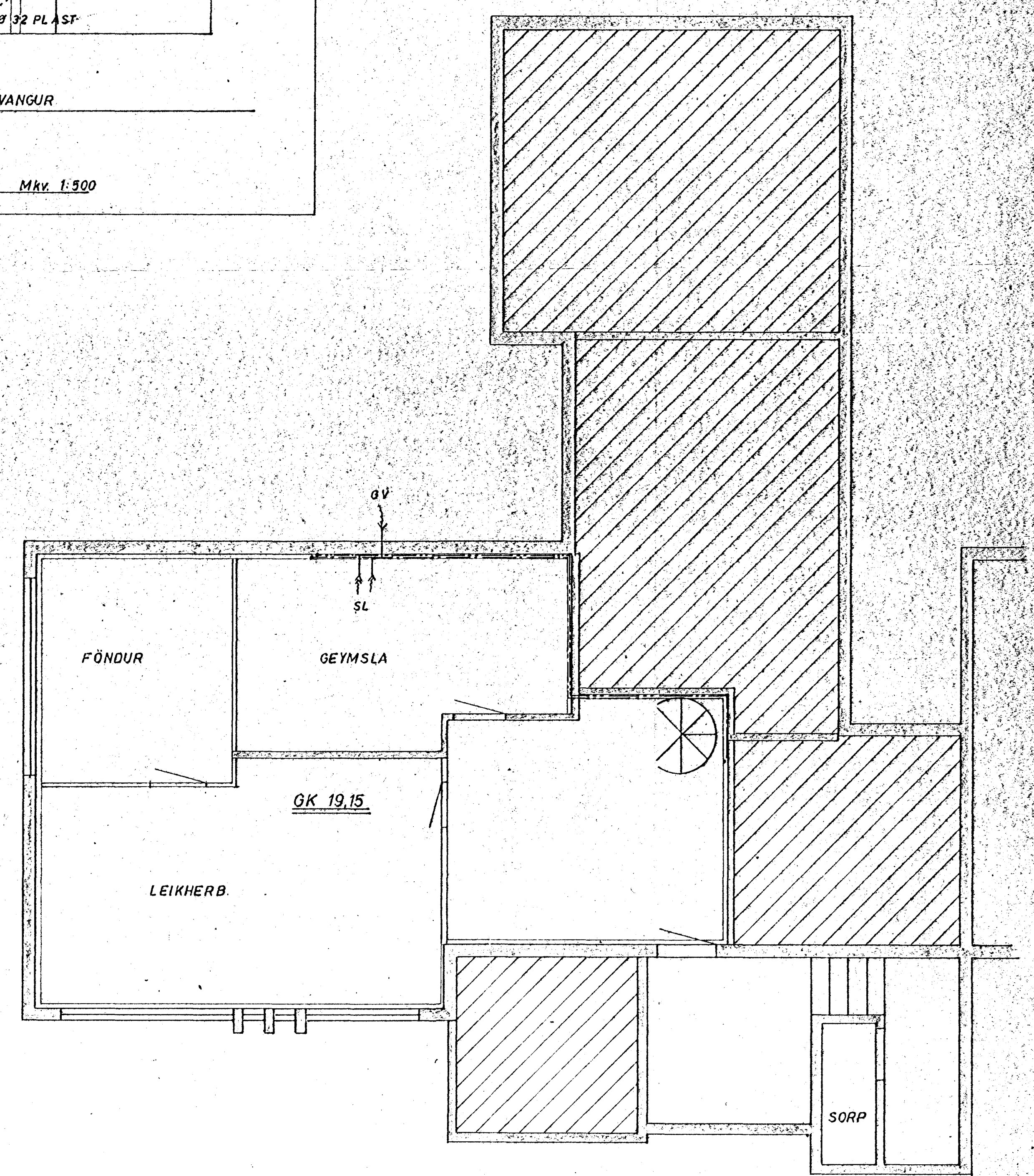
GRUNNMYND KJALLARA MKV. 1:50
