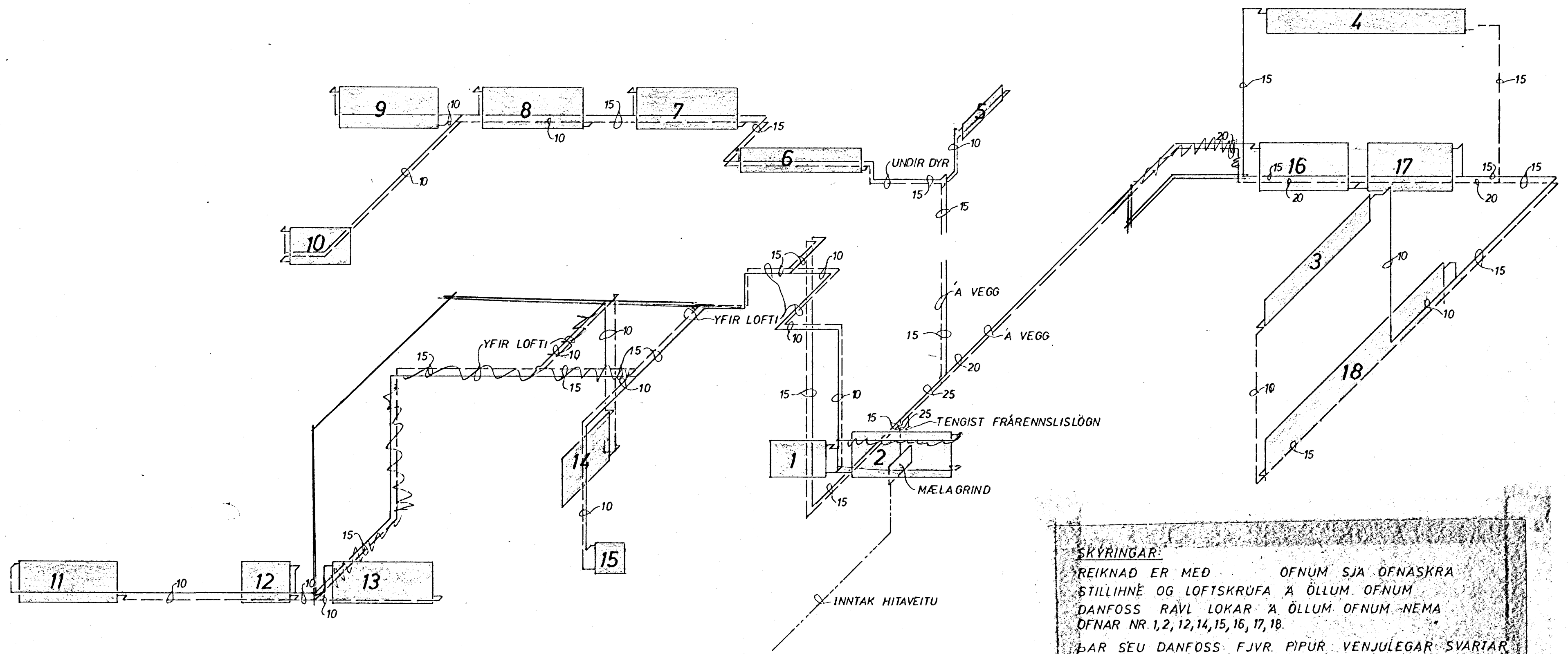
KERFI ~1:50
